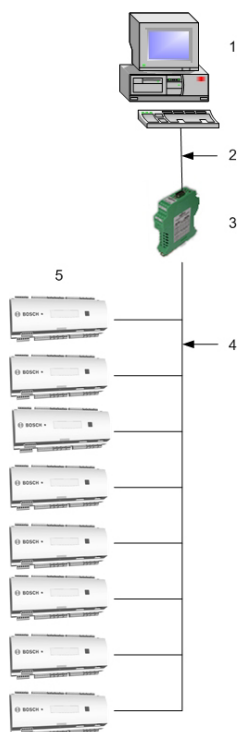
Рис. 4.8: Настройка главной системы RS-485
