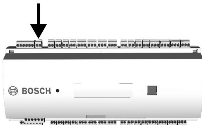
Рис. 4.20: Расположение контакта защиты от несанкционированного доступа
