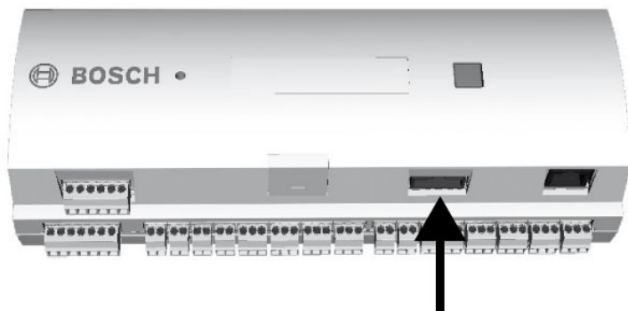
Рис. 4.11: Расположение последовательного интерфейса RS-232
