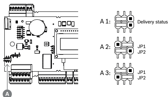
Рис. 4.5: Расположение перемычки заземления интерфейса главного компьютера RS-485
