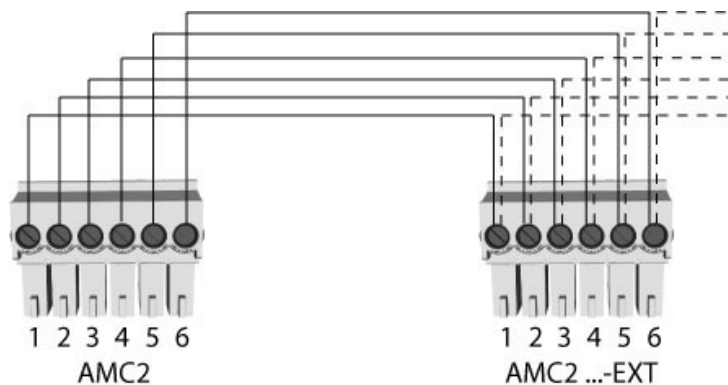
Рис. 4.14: Подключение модуля расширения к AMC2
