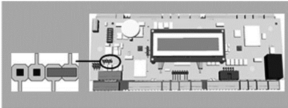
Рис. 4.9: Настройка перемычек для двухпроводных подключений RS-485
