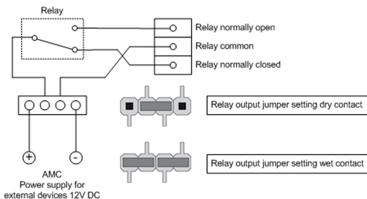
Рис. 4.16: Влажный режим и сухой режим релейных выходов AMC2
