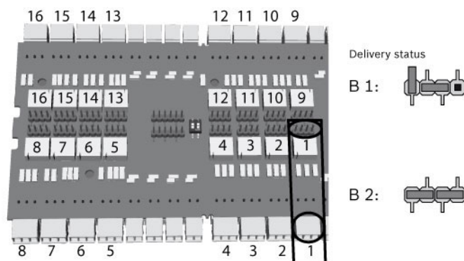
Рис. 4.18: Расположение перемычек релейных выходов
