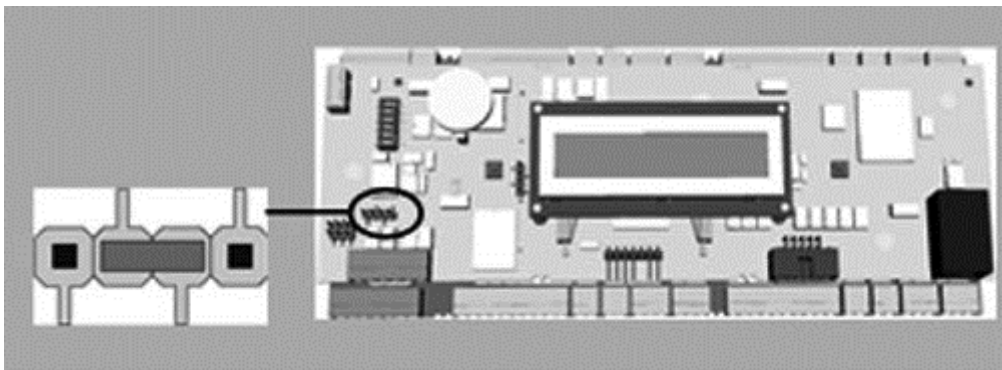
Рис. 4.10: Настройки для четырехпроводного подключения RS-485
