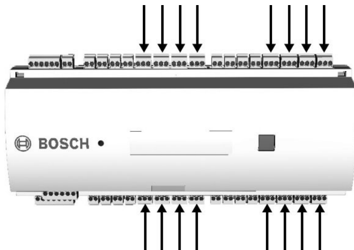
Рис. 4.15: Расположение разъемов релейных выходов
