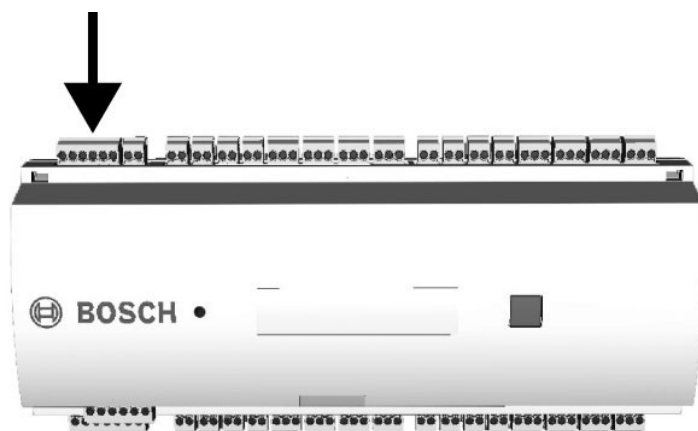
Рис. 4.13: Расположение шины модуля расширений RS-485
