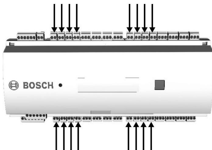
Рис. 4.19: Расположение разъемов аналоговых входов
