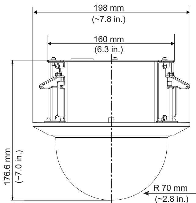
Infälld takmontering
