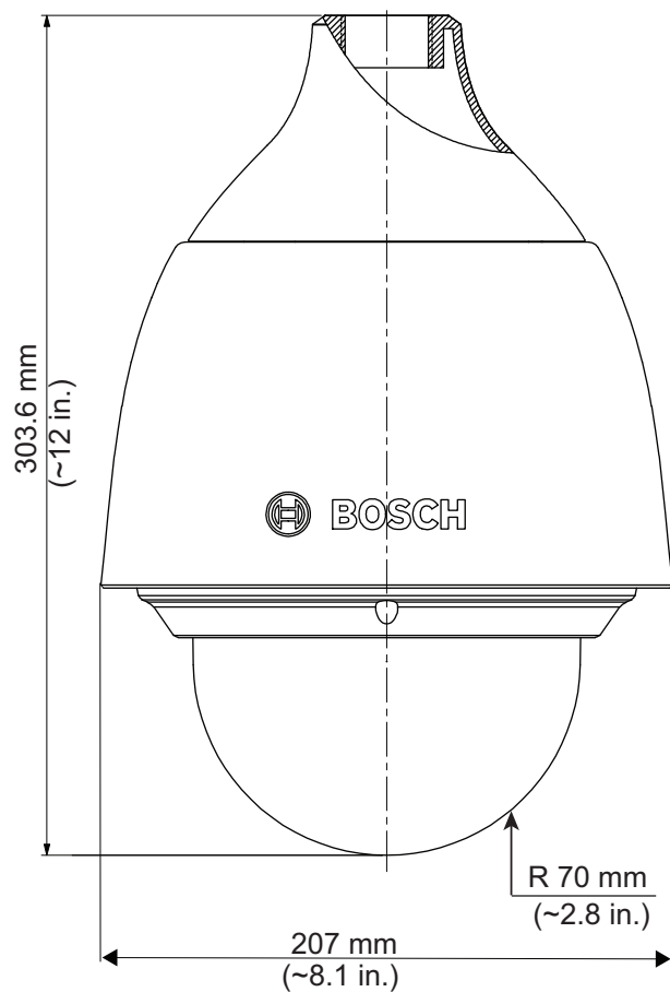
室外吊装型号
