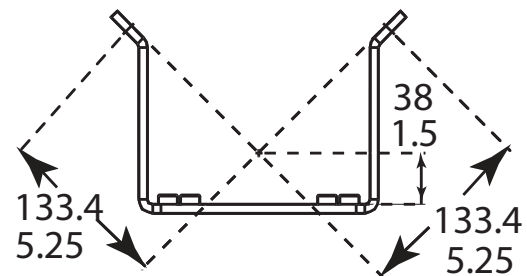
VG4-A-9541_立杆式安装适配器_尺寸
