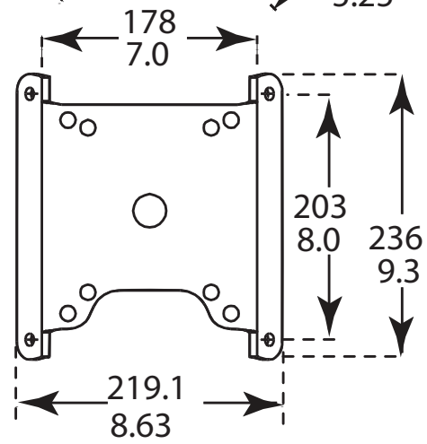
VG4-A-9542_墙角安装适配器_尺寸
