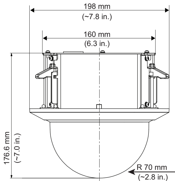
嵌入天花板式型号
