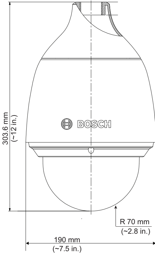
室内吊装式型号
