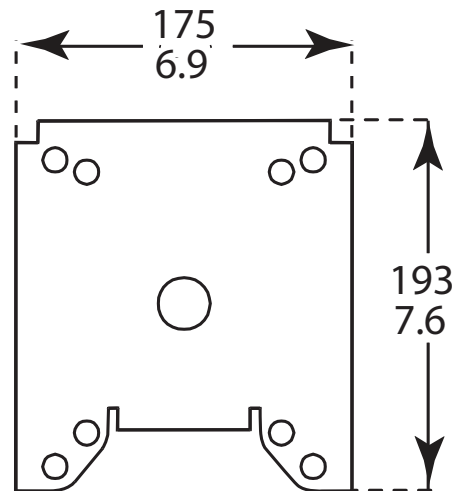
VG4-A-9541_立杆式安装适配器_尺寸
