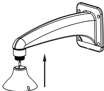
図 9.2: 壁面マウントへの取付キャップの取り付け
