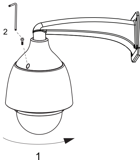
図 9.4: カメラのマウントへの固定
