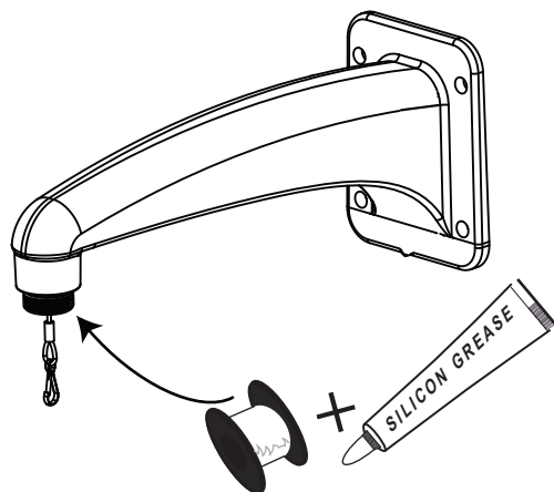
図 9.1: 壁面マウントのねじ山へのテープの巻き付けとグリースの塗布
