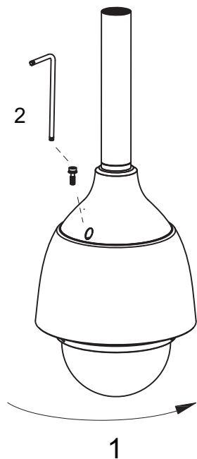
図 10.1: カメラのマウントへの固定
