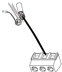
図 9.3: 壁面マウントのケーブル配線
