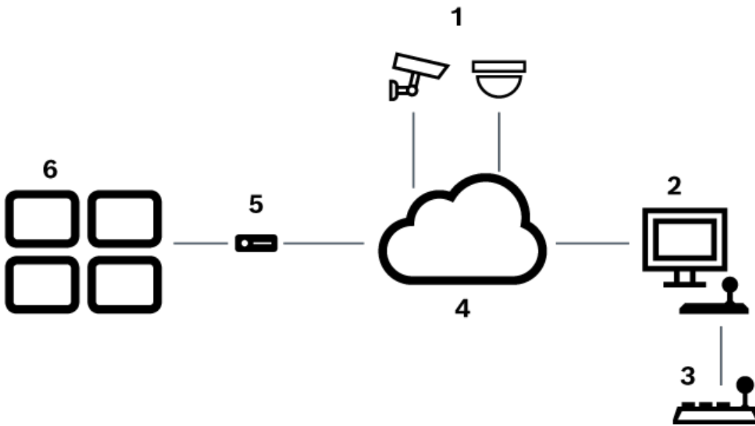
Figura 6.1: Scenario 1: utilizzo di una tastiera IntuiKey collegata ad una workstation BVMS
