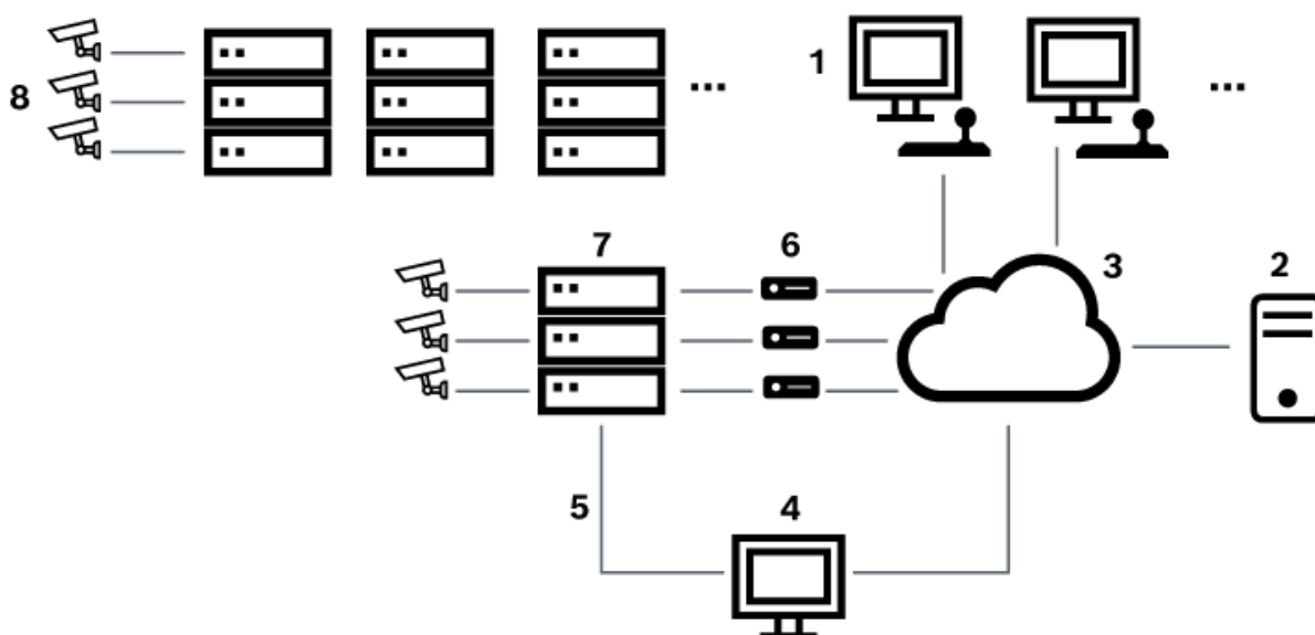
Figura 6.5: Sistema Allegiant esteso con commutatori satellitari
