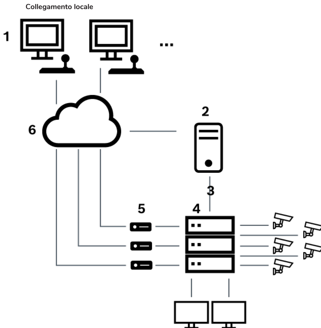
Figura 6.3: Collegamento locale di BVMS ad una matrice Allegiant
