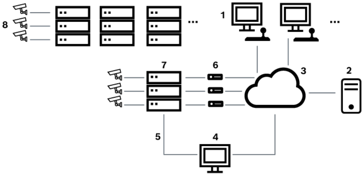
Attēls 6.5: Allegiant sistēma, kas paplašināta ar satelīta slēdžiem
