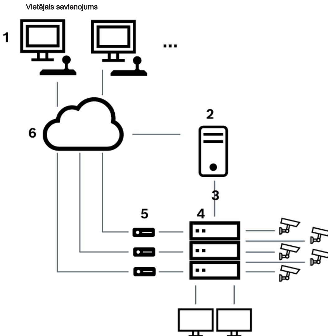
Attēls 6.3: BVMS lokālais savienojums ar Allegiant matricas slēdži
