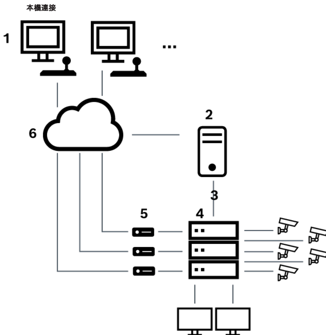
圖片 6.3: BVMS 本機連接至 Allegiant 矩陣切換器
