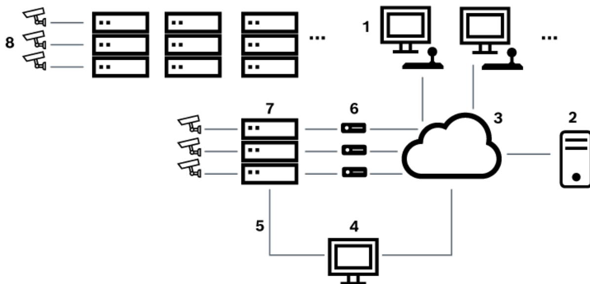
圖片 6.5: 以 Satellite 交換器延伸的 Allegiant 系統
