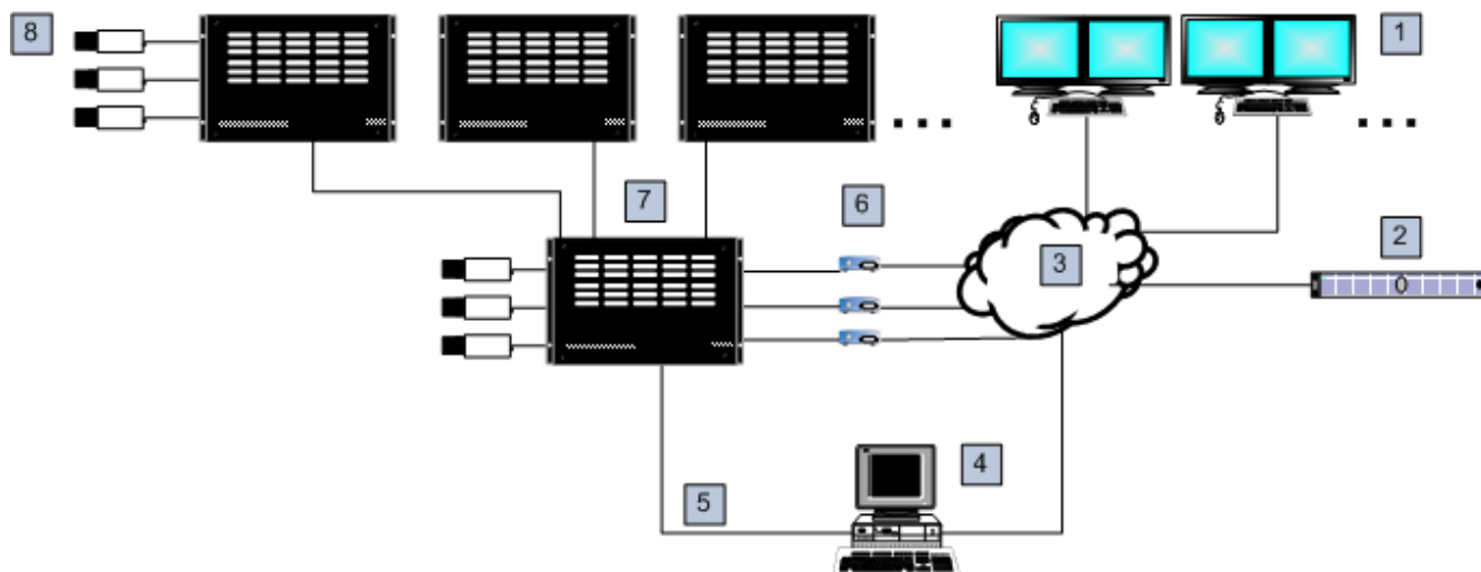
Σχήμα 5.5: Σύστημα Bosch Allegiant επεκτεταμένο με μεταγωγείς Satellite
