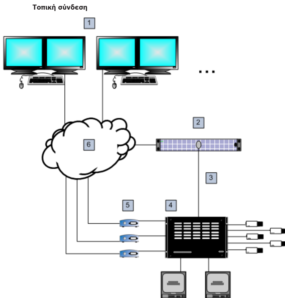
Σχήμα 5.3: Τοπική σύνδεση του Bosch Video Management System με μεταγωγέα συσκευής μητρώου Allegiant της Bosch
