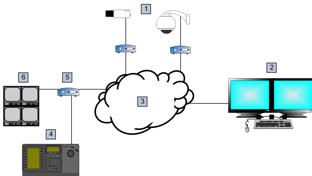
Σχήμα 5.2: Σενάριο 2: Πληκτρολόγιο IntuiKey της Bosch συνδεδεμένο με αποκωδικοποιητή
