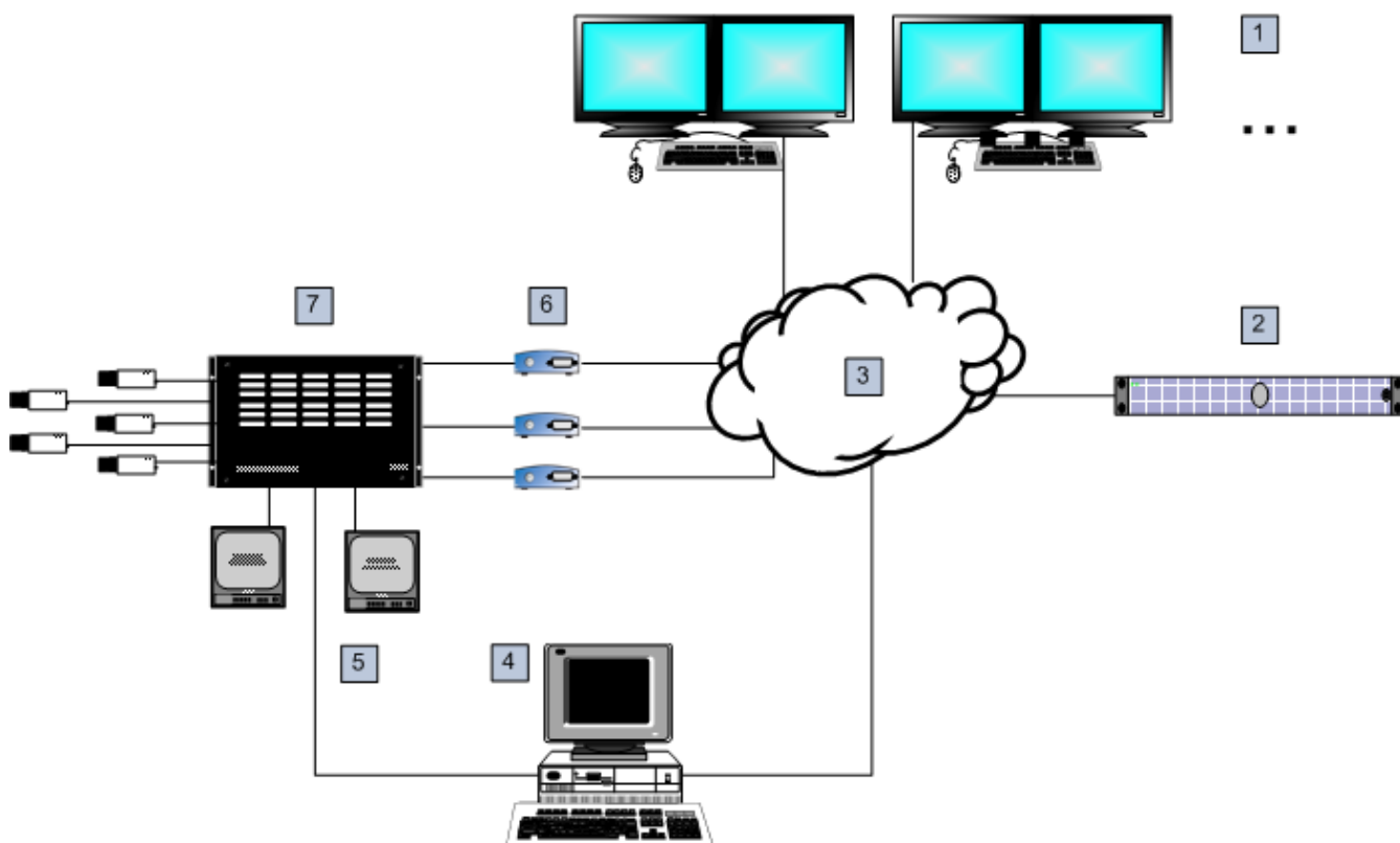
Σχήμα 5.4: Απομακρυσμένη σύνδεση του Bosch Video Management System με μεταγωγέα συσκευής μητρώου Allegiant της Bosch
