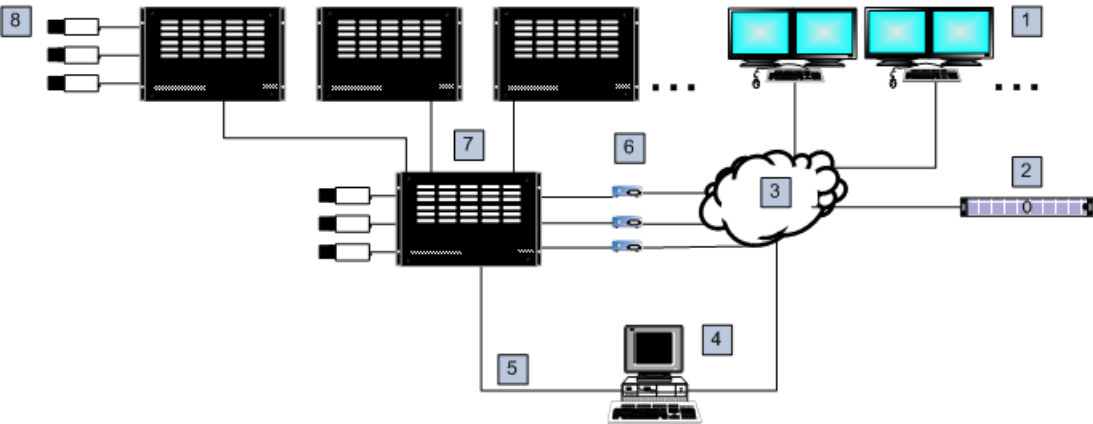
Figure 5.8: Système Bosch Allegiant étendu à l'aide de systèmes de commutation satellites
