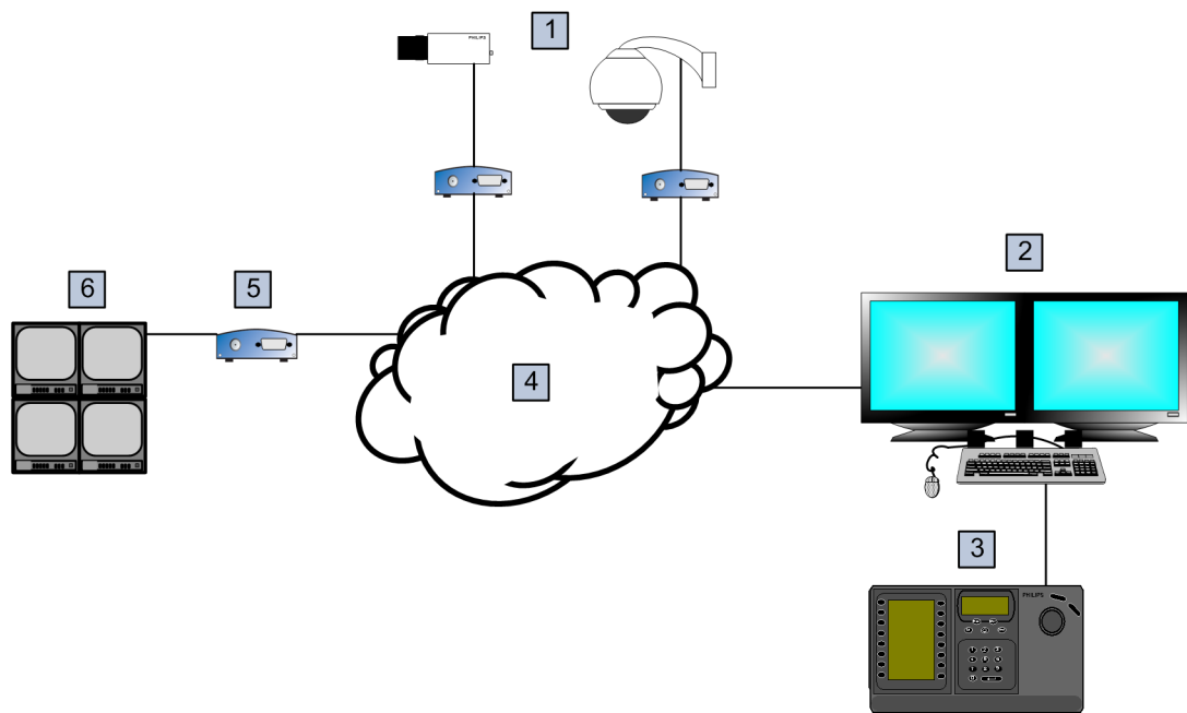
Figure 5.4: Scénario 1 : clavier numérique IntuiKey de Bosch connecté à un poste de commande Bosch Video Management System
