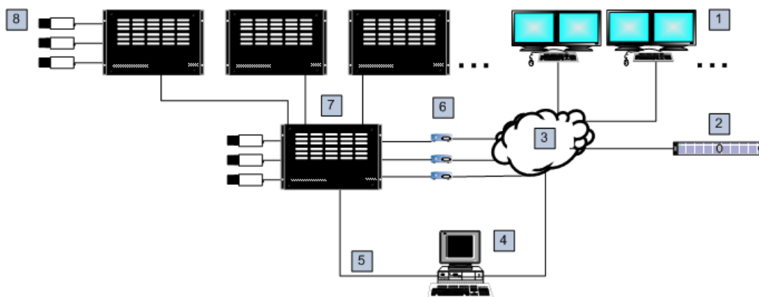
Figura 5.8: Sistema Bosch Allegiant esteso con commutatori satellitari
