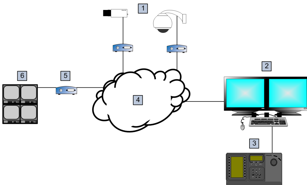
Rysunek 5.4: Sposób 1: klawiatura Bosch IntuiKey podłączona do stacji roboczej systemu Bosch Video Management System
