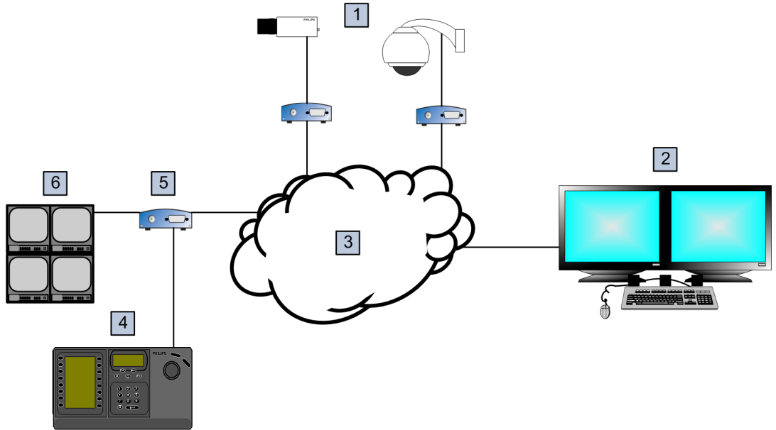
图 5.5: 方案 2 : Bosch IntuiKey 键盘连接到解码器
