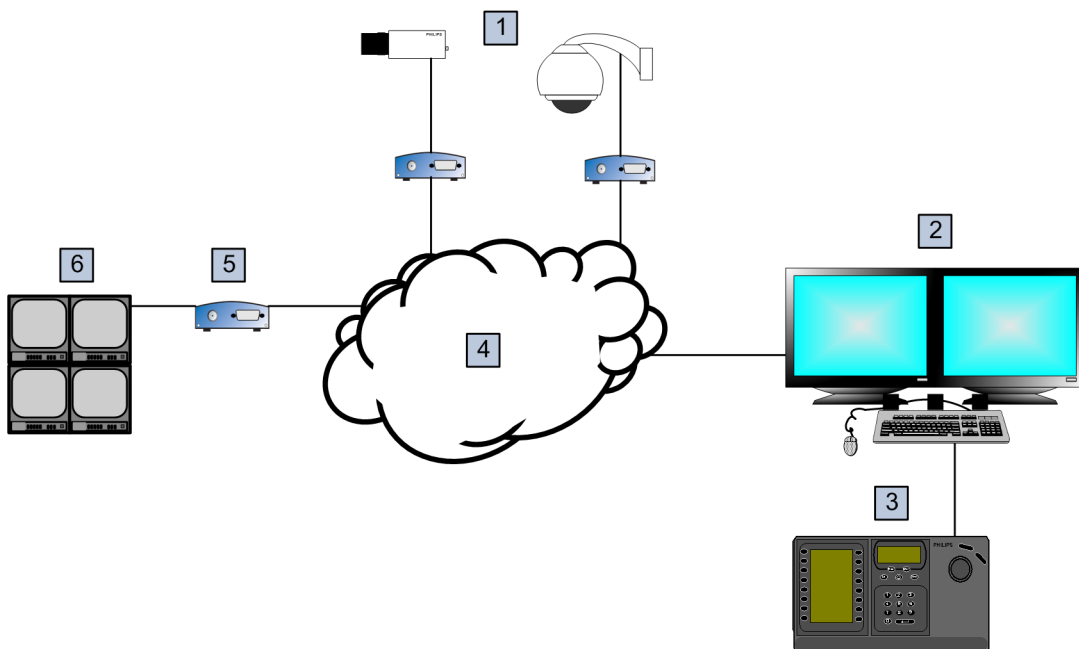
图 5.4: 方案 1 : Bosch IntuiKey 键盘连接到 Bosch Video Management System 工作站
