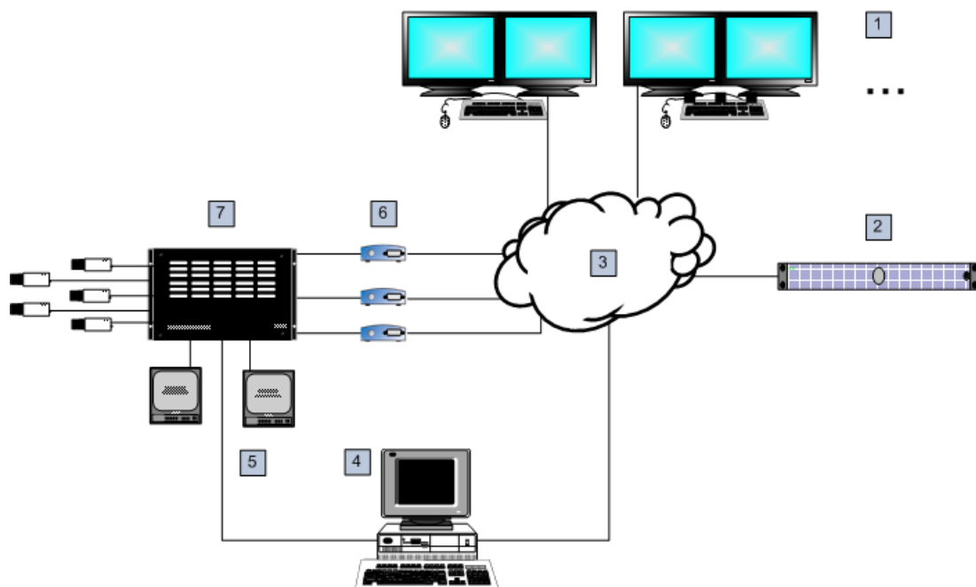
그림 5.1: Bosch Allegiant 매트릭스 스위치에 대한 Bosch Video Management System 원격 연결
