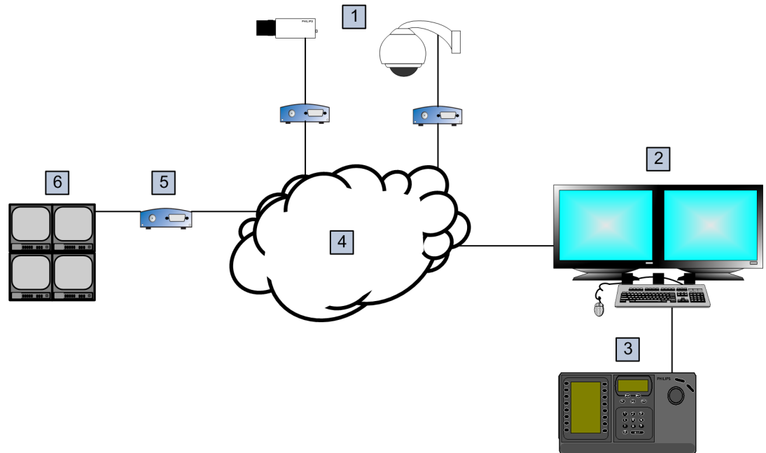
그림 5.1: 시나리오 1: Bosch Video Management System 워크스테이션에 연결된 Bosch IntuiKey 키보드
