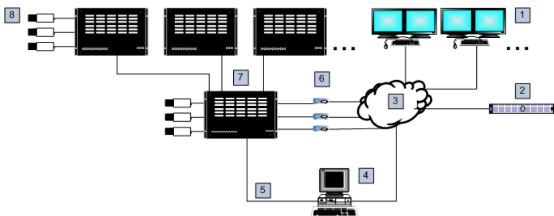
Рисунок 5.1: Система Bosch Allegiant, расширенная за счет сателлитных коммутаторов
