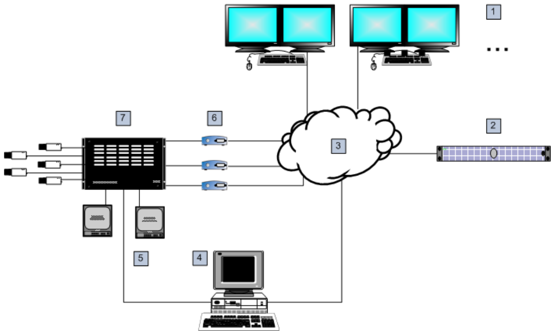
Рисунок 5.1: Удаленное подключение Bosch Video Management System к матричному коммутатору Bosch Allegiant
