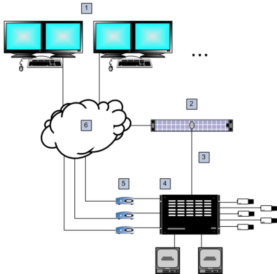
Рисунок 5.1: Локальное подключение Bosch Video Management System к матричному коммутатору Bosch Allegiant
