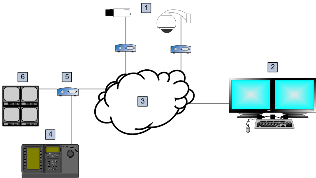
Рисунок 5.1: Сценарий 2: клавиатура Bosch IntuiKey, подключенная к декодеру
