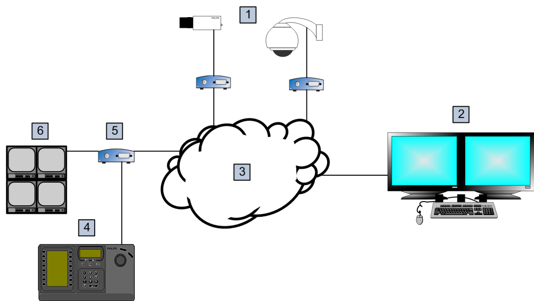
圖形 5.1: 情境 2: 連接至解碼器的 Bosch IntuiKey 鍵盤
