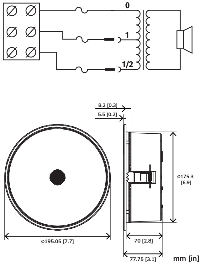
Fig. 1: Dimensions
