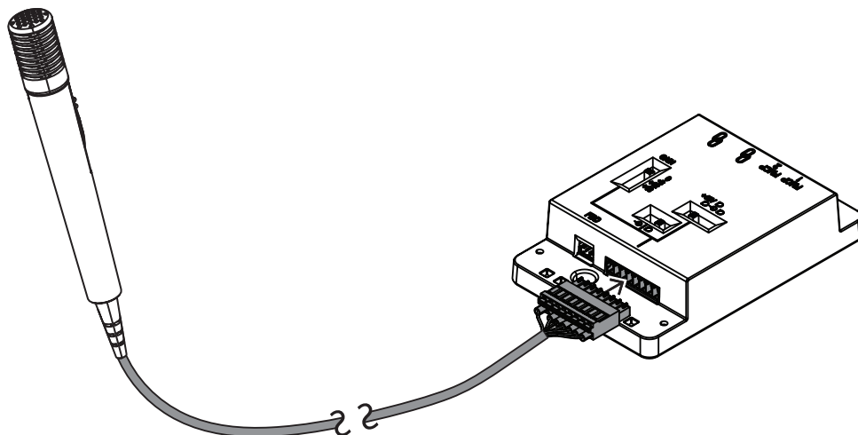
Abbildung 7.17: Das DCNM-FAI mit dem DCNM-FHH / DCNM-FHHC verbinden
