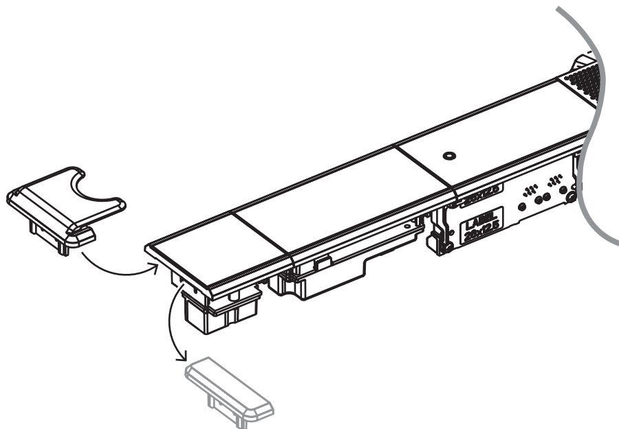
Abbildung 7.20: Den DCNM-FEC durch den DCNM-FICH ersetzen
