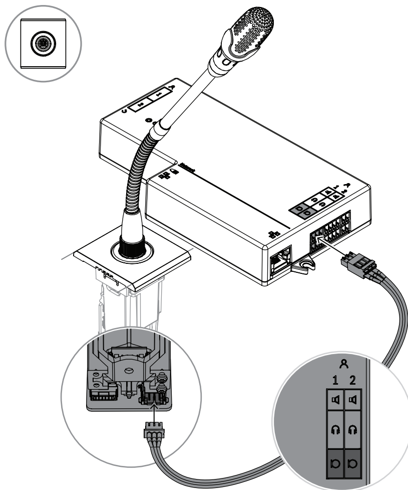
Abbildung 7.5: Anschließen des DCNM-FMCP an die DCNM-FBD2
