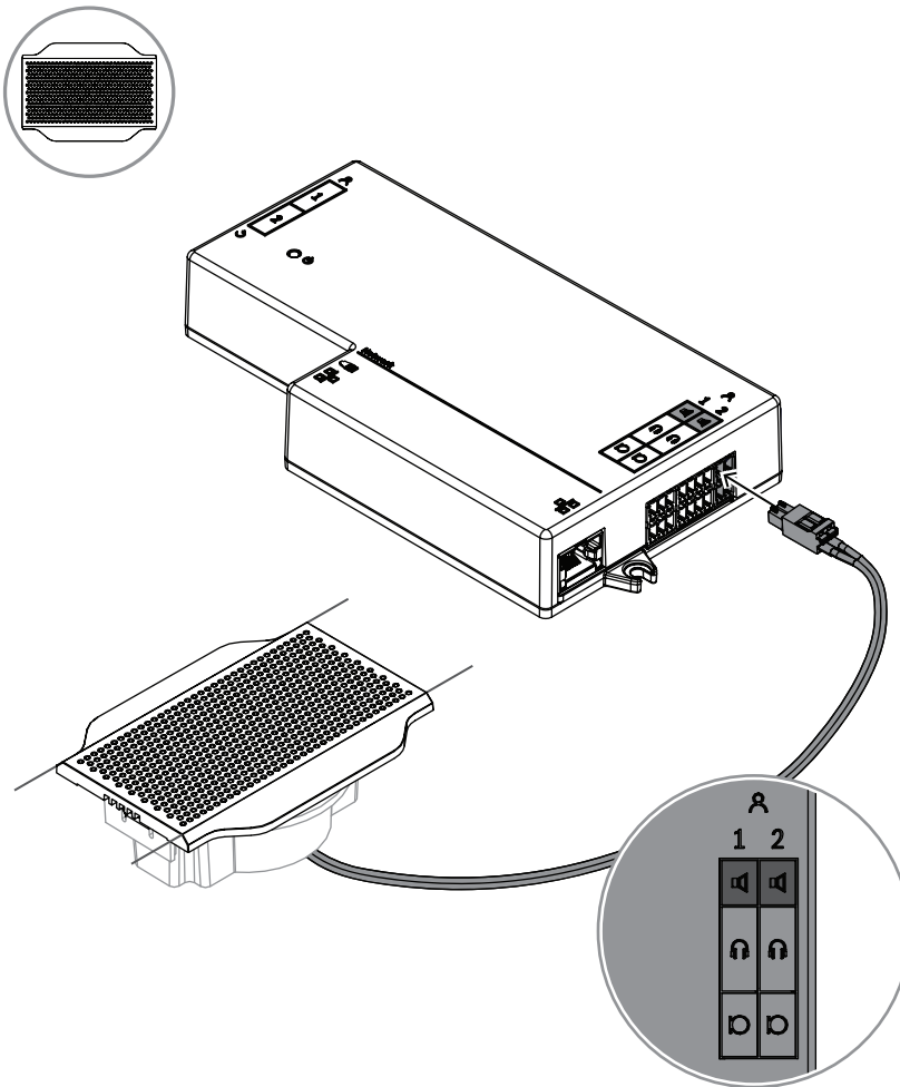
Abbildung 7.6: Anschließen eines DCNM-FLSP an die DCNM-FBD2
