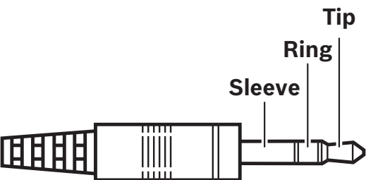
Abbildung 7.14: Kopfhörerbuchsenanschluss
