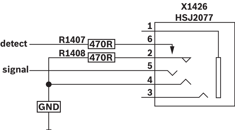
Abbildung 7.13: Schema für externen Kopfhöreranschluss
