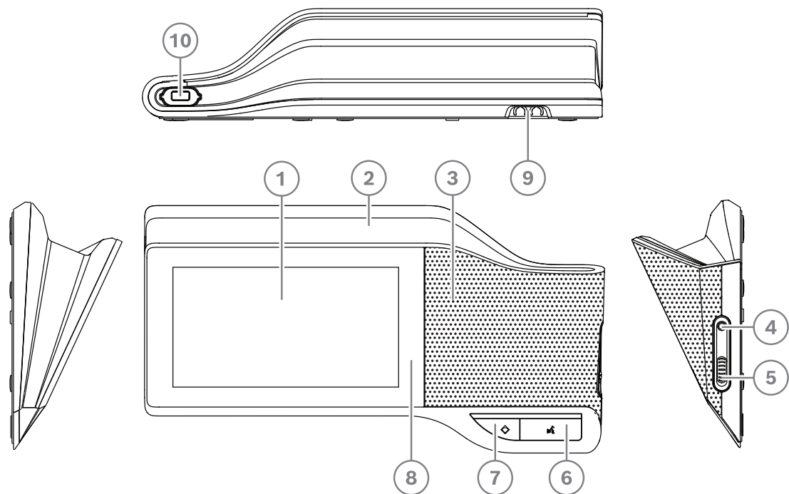
Abbildung 7.1: Frontansicht, Draufsicht, Rück- und Seitenansicht
