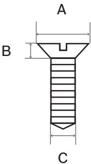
Abbildung 5.13: Max. Abmessungen der Schrauben
