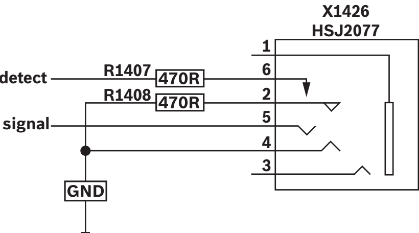
Abbildung 7.23: Schema für externen Kopfhöreranschluss
