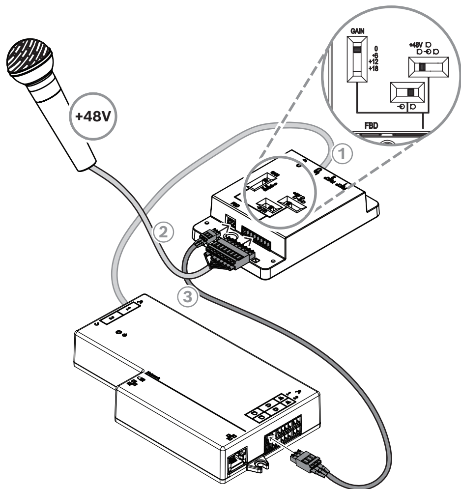
Abbildung 7.16: Anschluss eines phantomgespeisten Mikrofons an die DCNM-FBD2 über das DCNM-FAI
