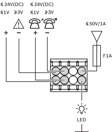
Abbildung 5.15: Anschlussdiagramm
