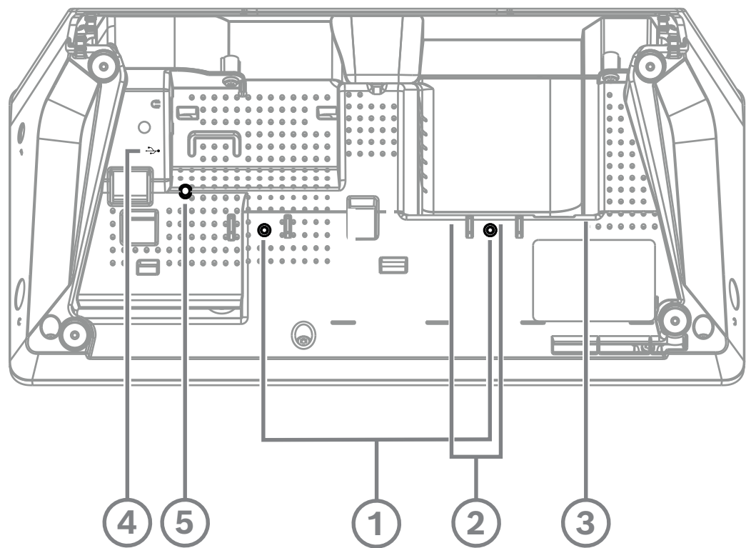
Abbildung 7.25: DCNM-IDE SK / DCNM-IDE SKVID Unteransicht
