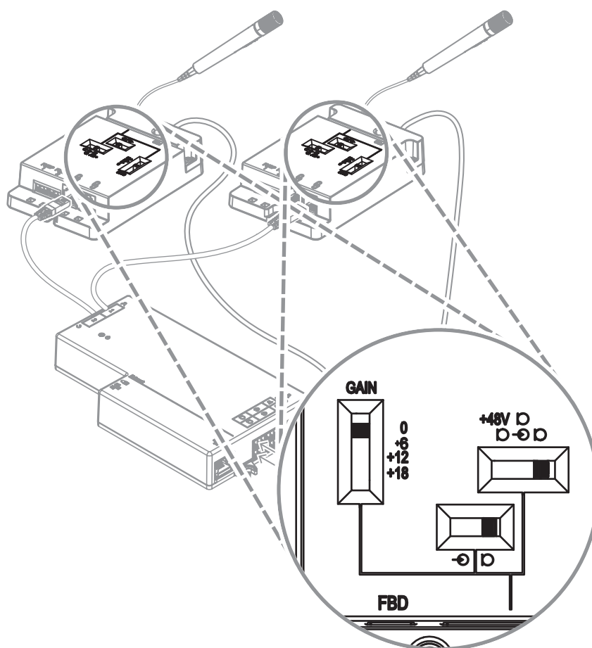
Abbildung 7.18: DCNM-FAI Schaltereinstellungen zum Anschluss des DCNM-FHH / DCNM-FHHC
