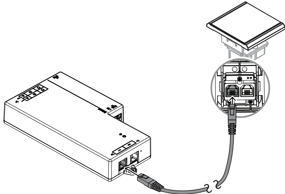
Abbildung 7.19: Das DCNM-FIDP zur Steuerung mit der DCNM-FBD2 verbinden
