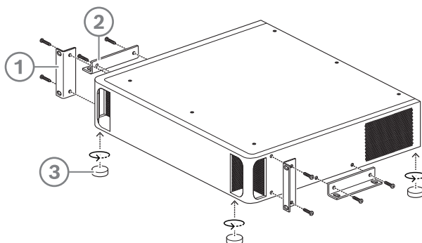
Abbildung 6.4: 19"-Rack-Montage, Tischmontage, Tischaufstellung mit Gerätefüßen
