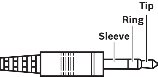
Abbildung 7.24: Kopfhörerbuchsenanschluss
