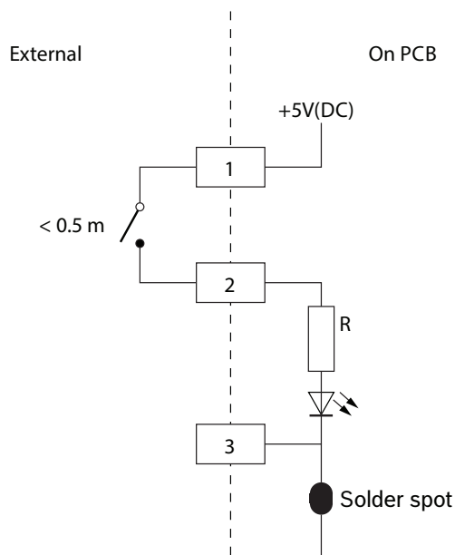
Abbildung 7.11: Externer Kontakt, Anschluss (2)
