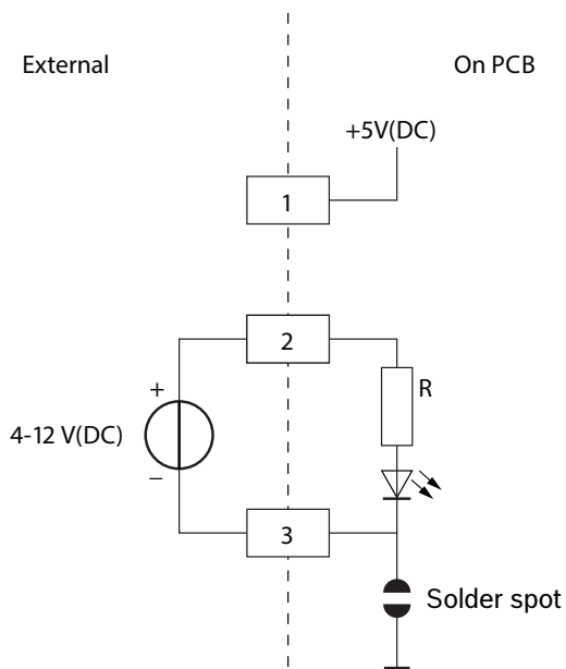
Abbildung 7.10: Externer Kontakt, Anschluss (1)
