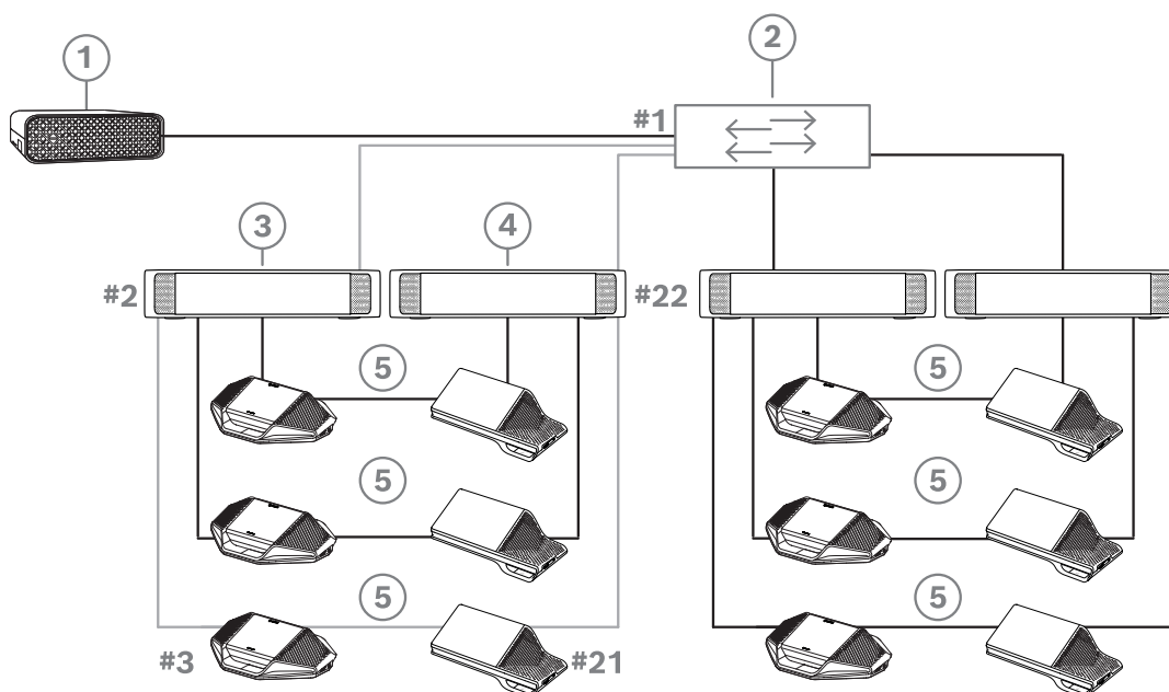
Abbildung 4.9: DICENTIS Diskussionseinheiten, die mit redundanter Verkabelung zwischen Einheiten vom Typ DCNM-PS2/DCNM-APS2 angeschlossen sind
