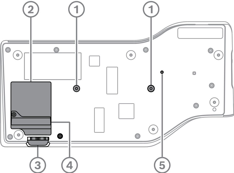
Abbildung 7.3: Unteransicht DICENTIS Diskussionseinheiten (DCNM-MMD/DCNM-MMD2)
