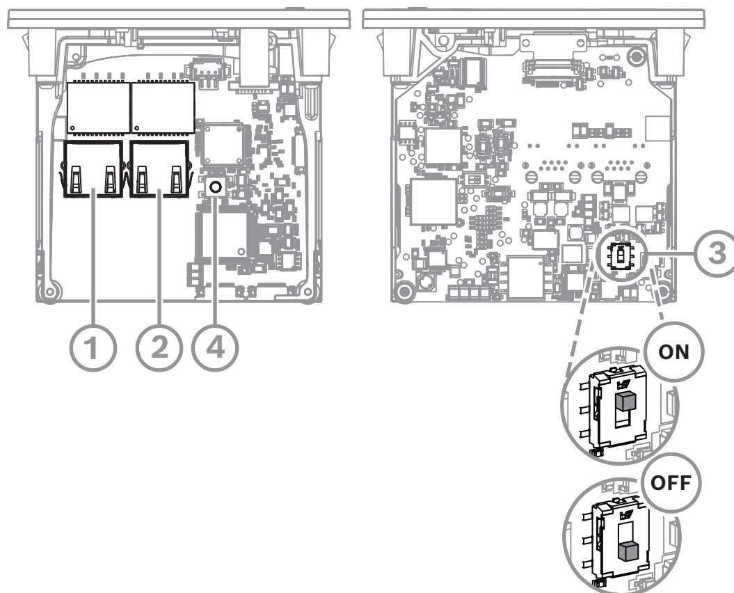
Abbildung 7.22: DCNM-FSL2
