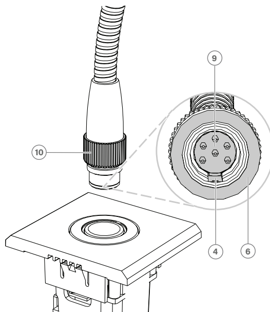
Abbildung 7.28: DCNM-MICSL / DCNM-MICSLS Anschluss
