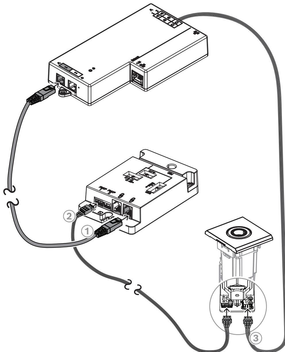
Abbildung 7.15: Anschluss des DCNM-FMCP an die DCNM-FBD2 über das DCNM-FAI
