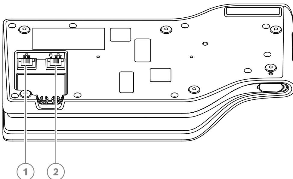
Abbildung 4.6: Unteransicht DICENTIS Einheiten (DCNM-MMD/DCNM-MMD2)
