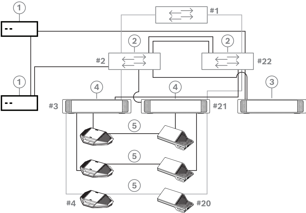
Abbildung 4.10: Redundante DICENTIS Server-PCs mit redundanten Komponenten und Kabeln
