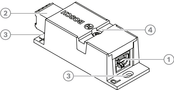
Abbildung 5.12: DCNM-IDE SKINT
