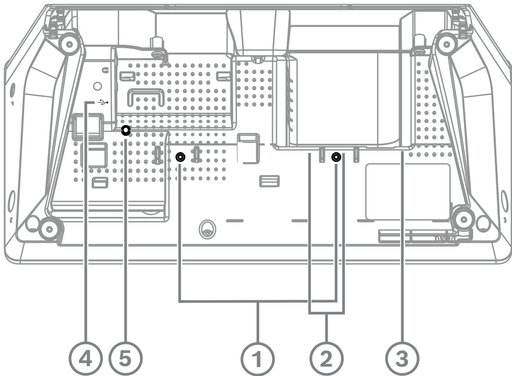
Figura 7.25: Vista inferior de DCNM-IDEK / DCNM-IDEKVID
