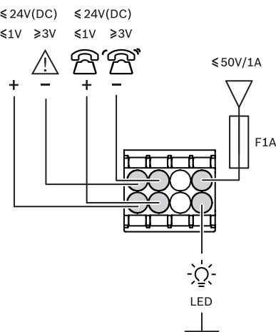
Figura 5.15: Diagrama de conexiones
