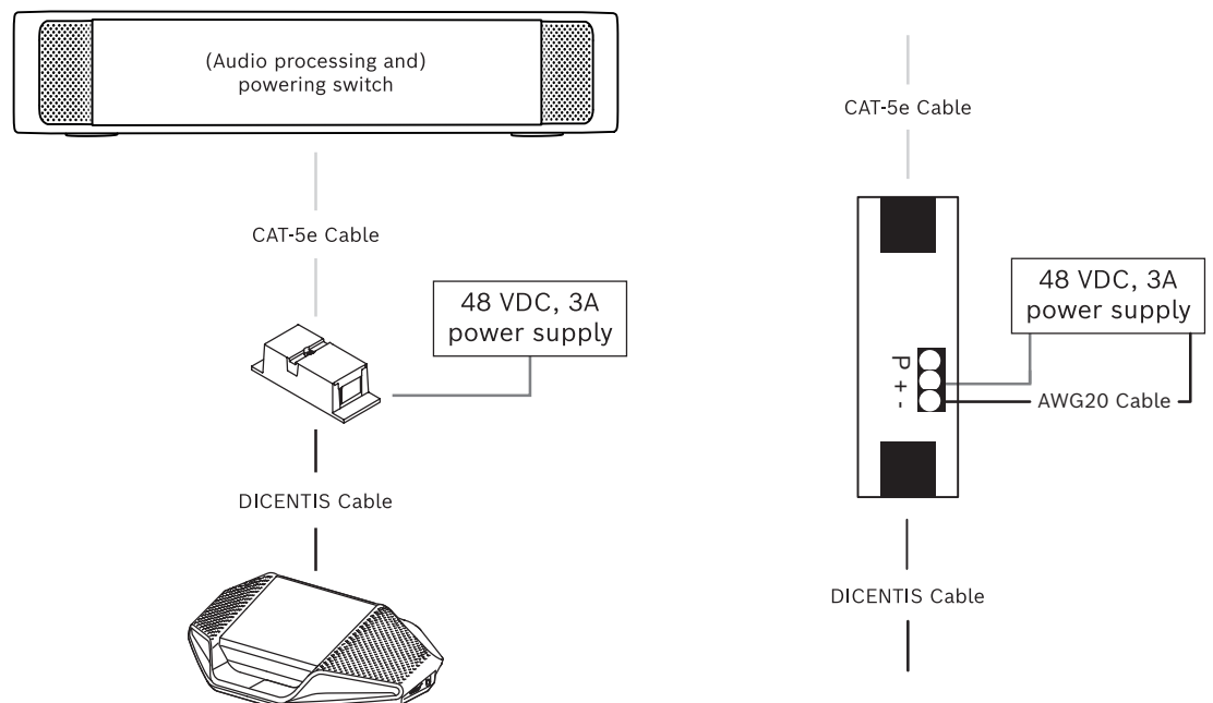
Figura 5.5: Conducción de la alimentación a través de cable
