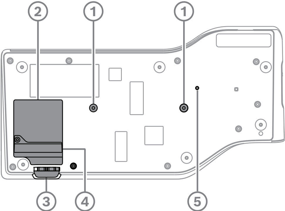
Figura 7.3: Vista inferior de los dispositivos de debate DICENTIS (DCNM-MMD / DCNM-MMD2)
