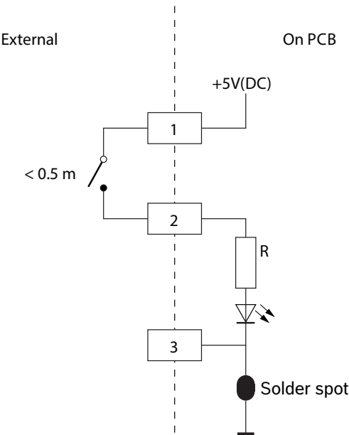
Figura 7.11: Contacto externo, conexión (2)
