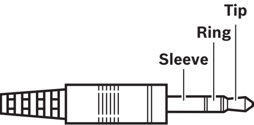
Figura 7.24: Collegamento jack cuffia
