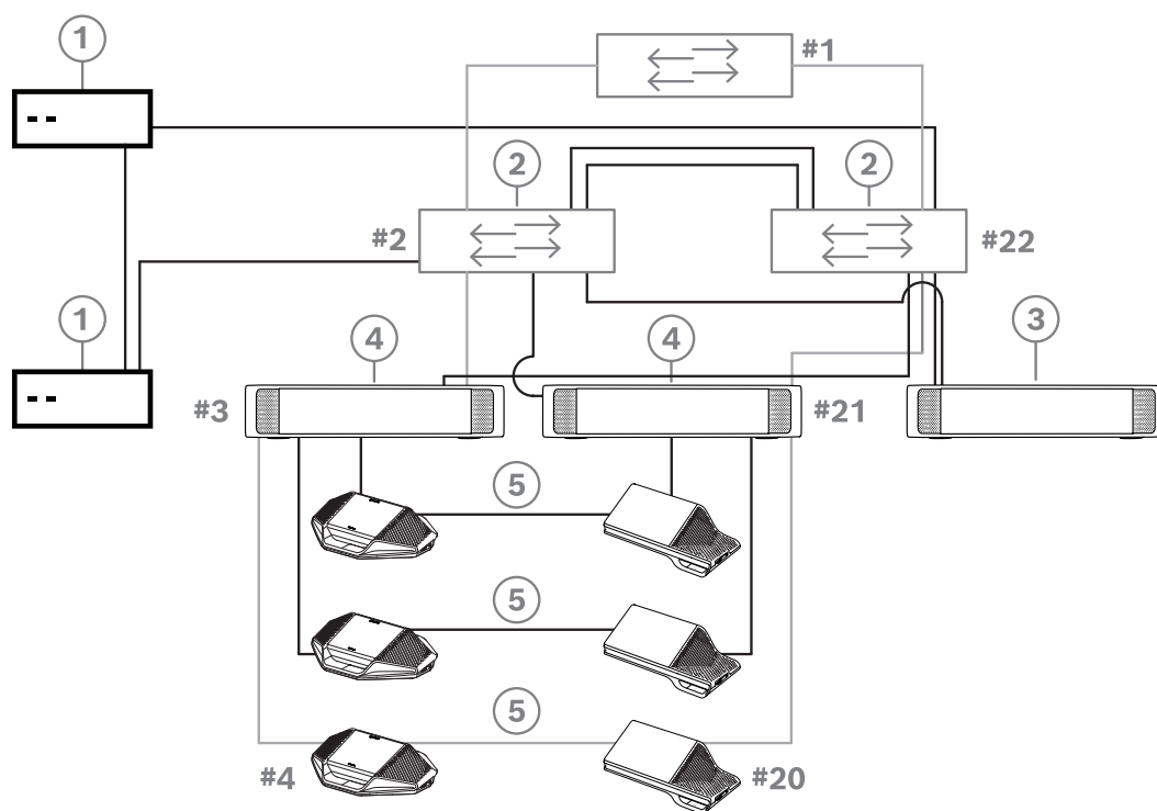
Figura 4.10: PC server DICENTIS ridondante con cavi e componenti ridondanti
