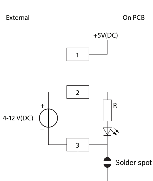
Figura 7.10: Contatto esterno, connessioni (1)
