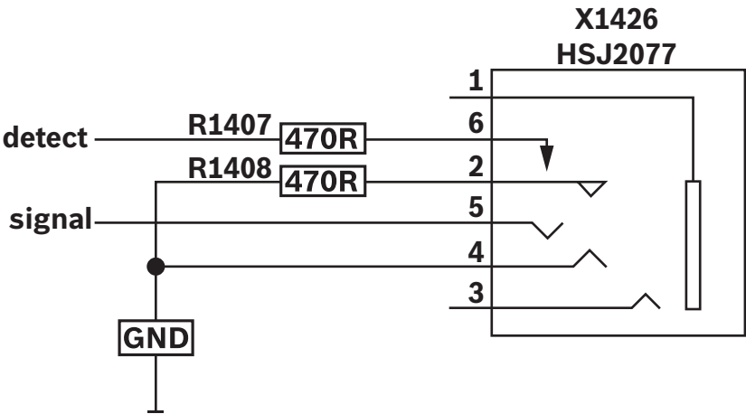
Figura 7.13: Schema connettore cuffia esterna
