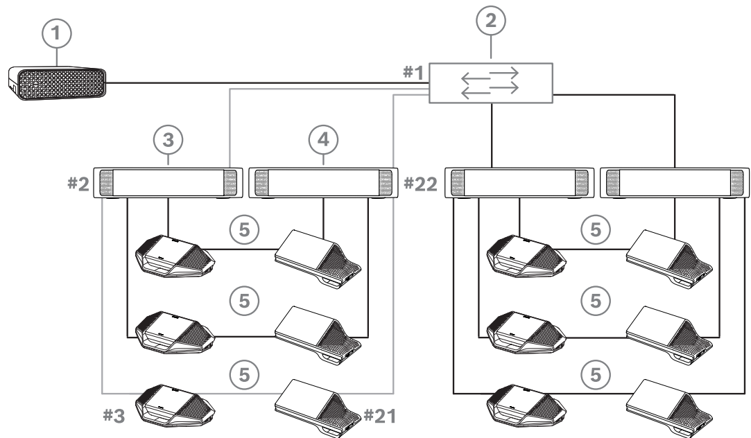
Figura 4.9: Dispositivi per dibattiti DICENTIS collegati con cavi ridondanti tra unità di tipo DCNM-PS2/DCNM-APS2
