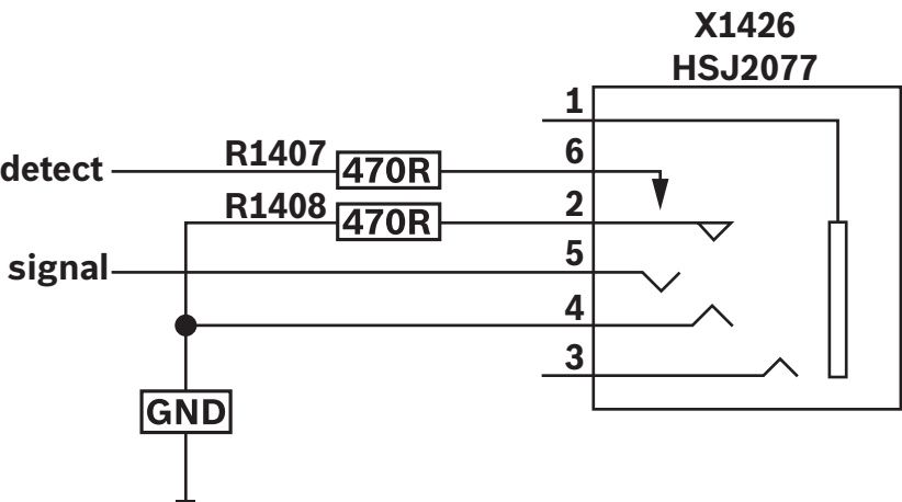
Figura 7.23: Schema connettore cuffia esterna
