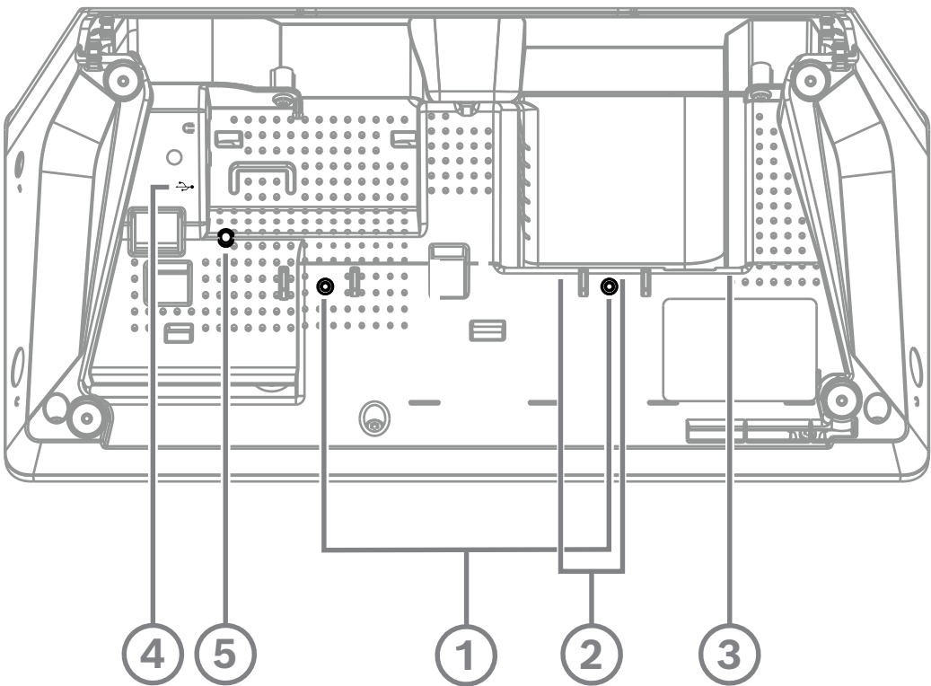
Figura 7.25: Vista dal basso di DCNM-IDE SK / DCNM-IDE SKVID
