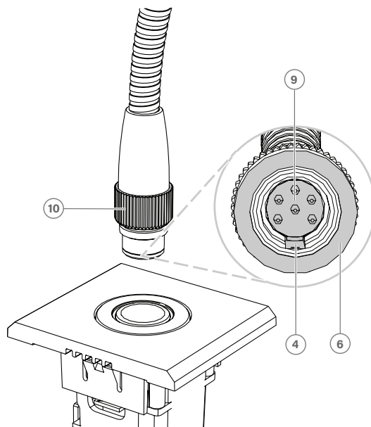
Figura 7.28: Collegamento di DCNM-MICSL/DCNM-MICSL
