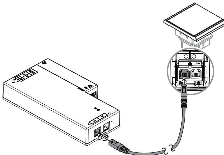
Figura 7.19: Collegare DCNM-FIDP a DCNM-FBD2 per il controllo
