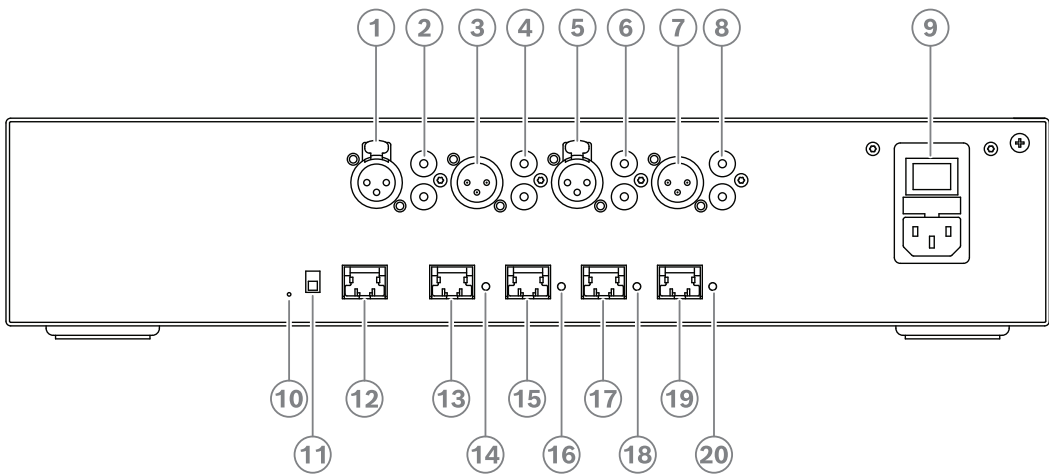
Figura 6.2: Switch di alimentazione e processo audio
