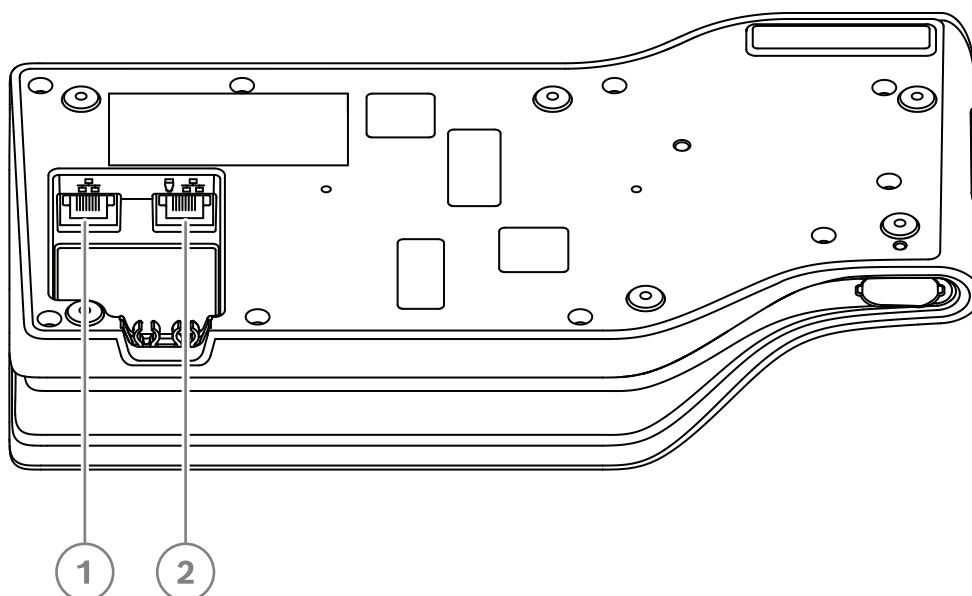
Figura 4.6: Vista dal basso, dispositivi DICENTIS (DCNM-MMD / DCNM-MMD2)
