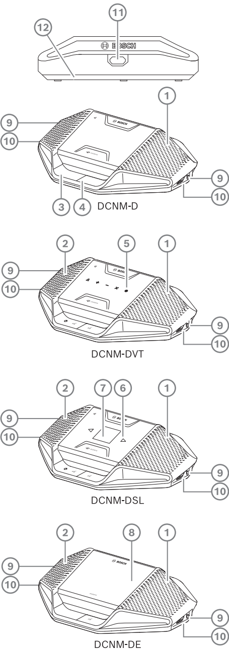
Figura 7.2: Viste anteriore, posteriore, laterale e dall'alto
