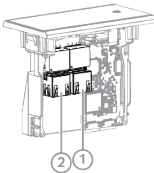
Figura 4.4: Vista dal basso di DCNM-FSL2
