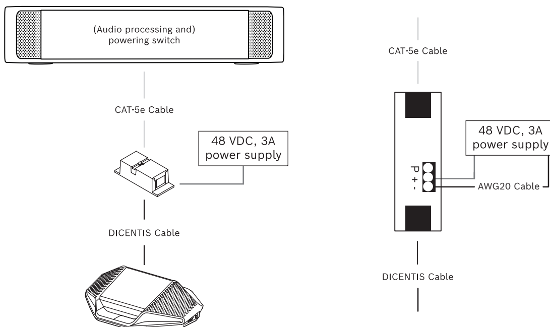
Figura 5.5: Trasporto dell'alimentazione via cavo
