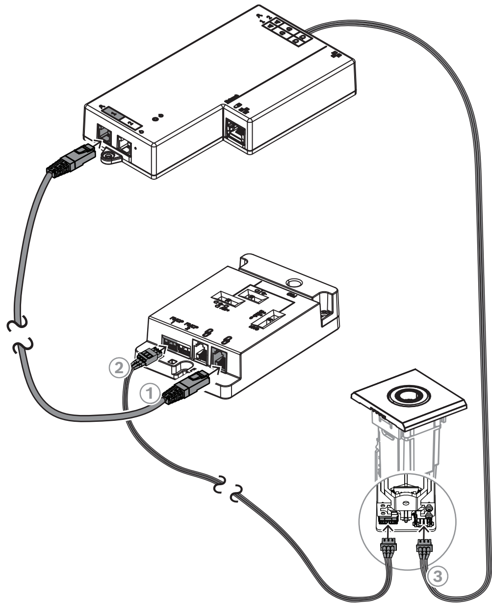
Figura 7.15: Collegare DCNM-FMCP a DCNM-FBD2 tramite DCNM-FAI
