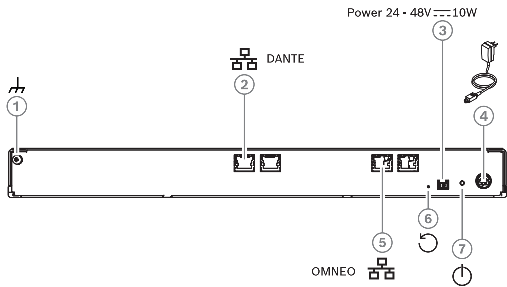
Figura 6.5: Descrizione del pannello posteriore di OMN-DANTEGTW
