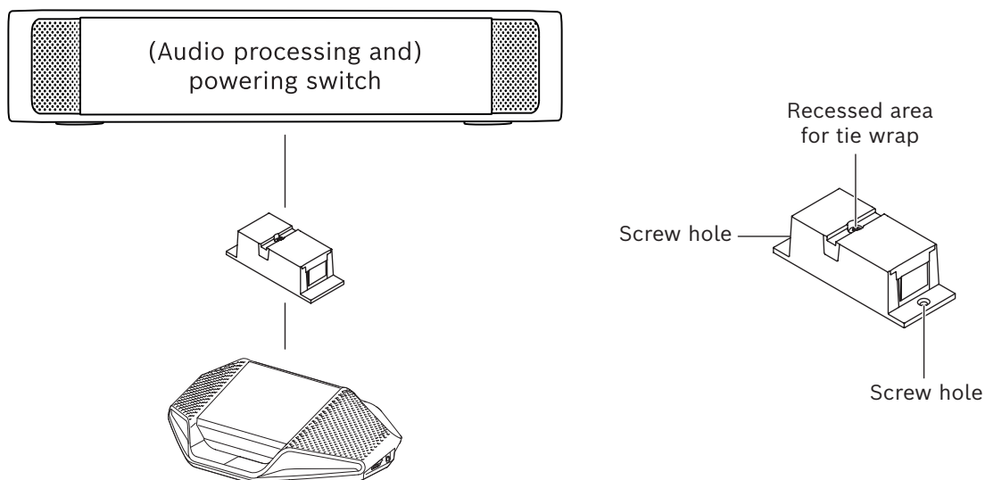
Figura 5.2: Installazione in una base da terra come breakout box
