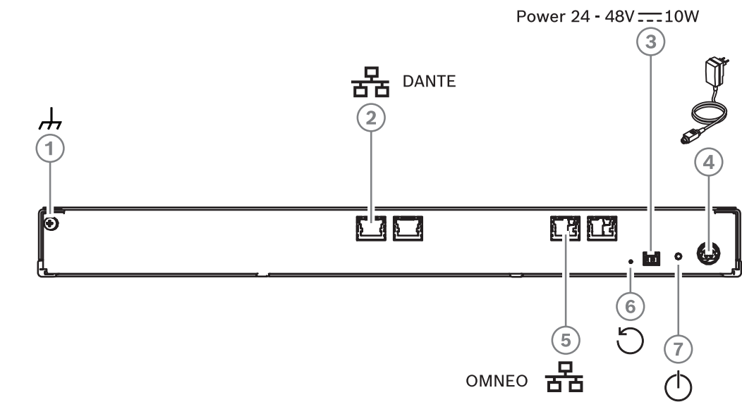
그림 6.5: OMN-DANTEGTW 후면 패널 설명
