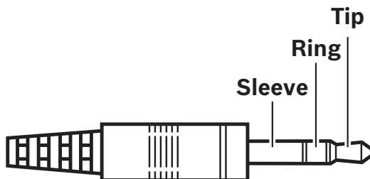
그림 7.14: 헤드폰 잭 연결
