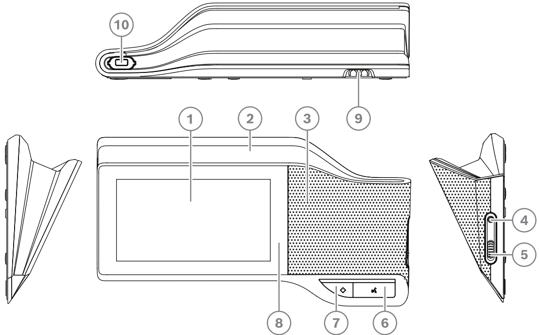
그림 7.1: 전면, 상단면, 후면, 측면
