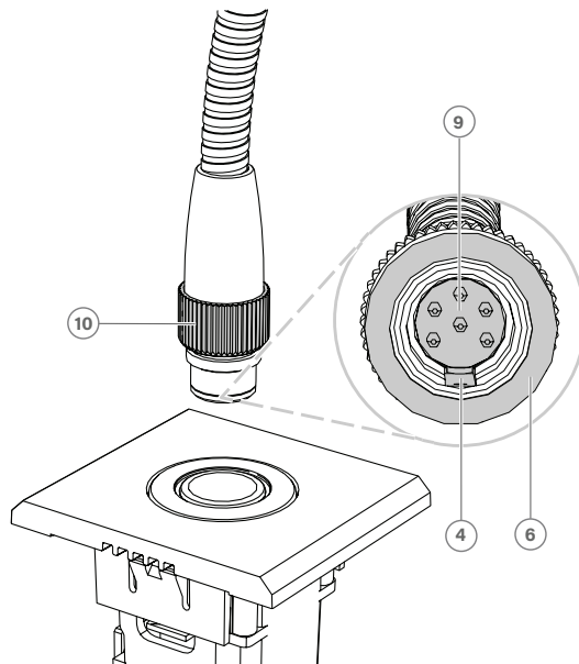
그림 7.28: DCNM-MICSL/DCNM-MICSLS 연결
