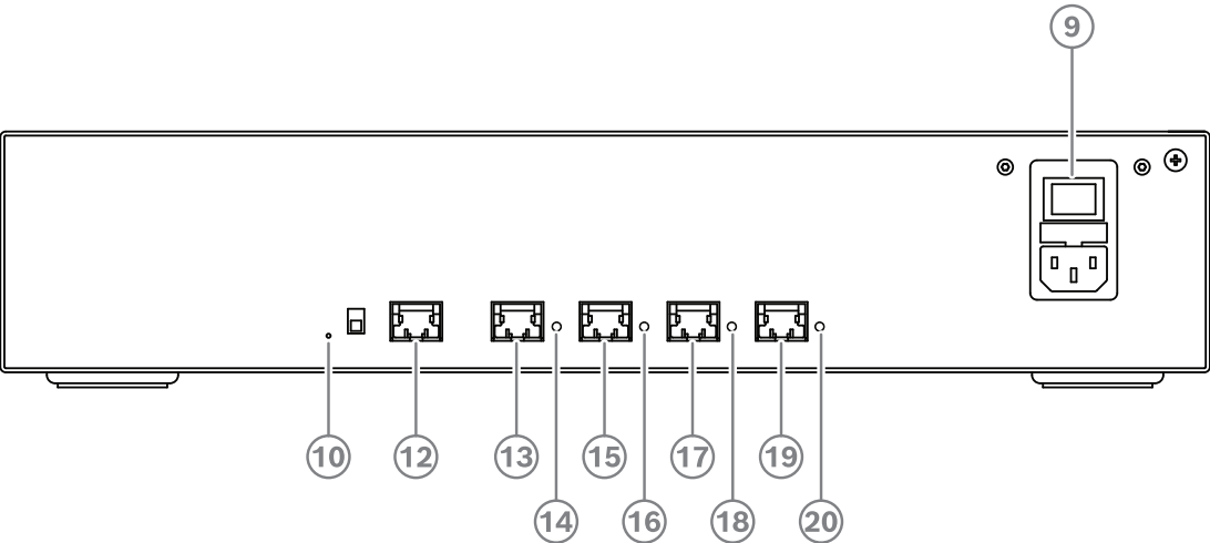
그림 6.3: 파워링 스위치
