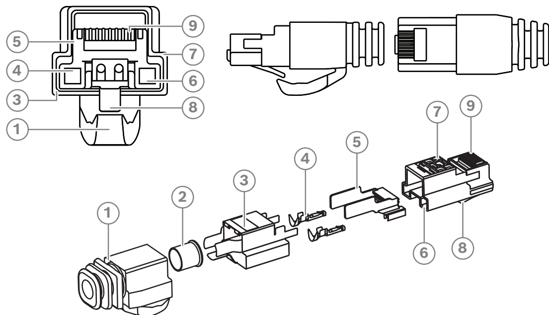
그림 5.10: DCNM-CBCON 전면 및 분해도
