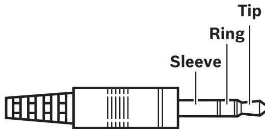
그림 7.24: 헤드폰 잭 연결
