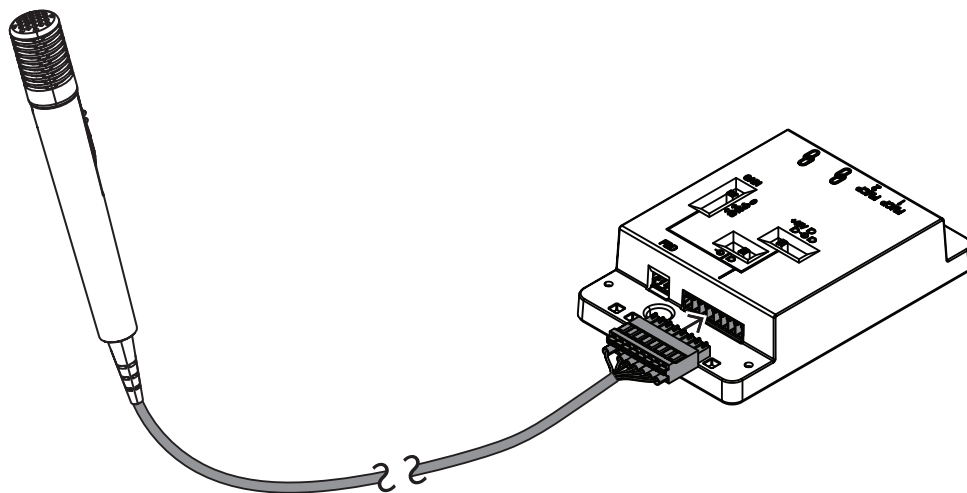
그림 7.17: DCNM-FAI를 DCNM-FHH/DCNM-FHHC에 연결
