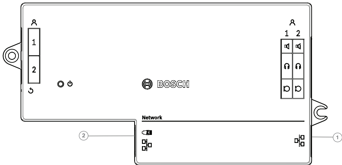
그림 4.8: 상단면 DICENTIS 매립형 베이스 장치(DCNM-FBD2)
