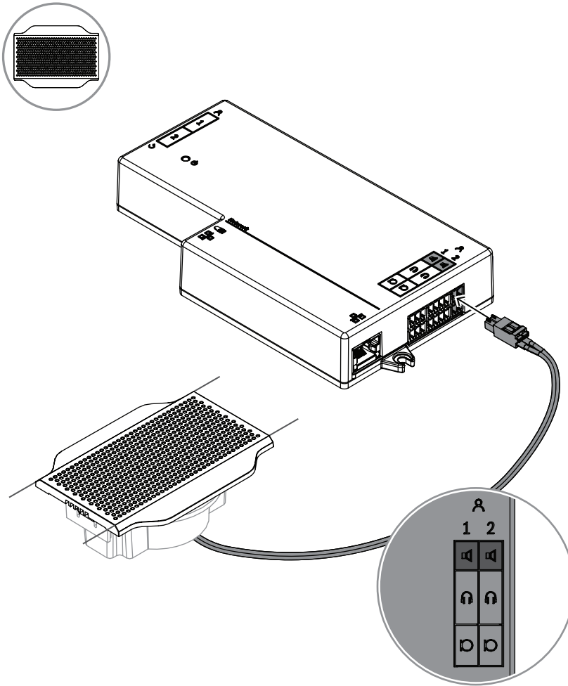
그림 7.6: DCNM-FBD2에 한 개의 DCNM-FLSP 연결
