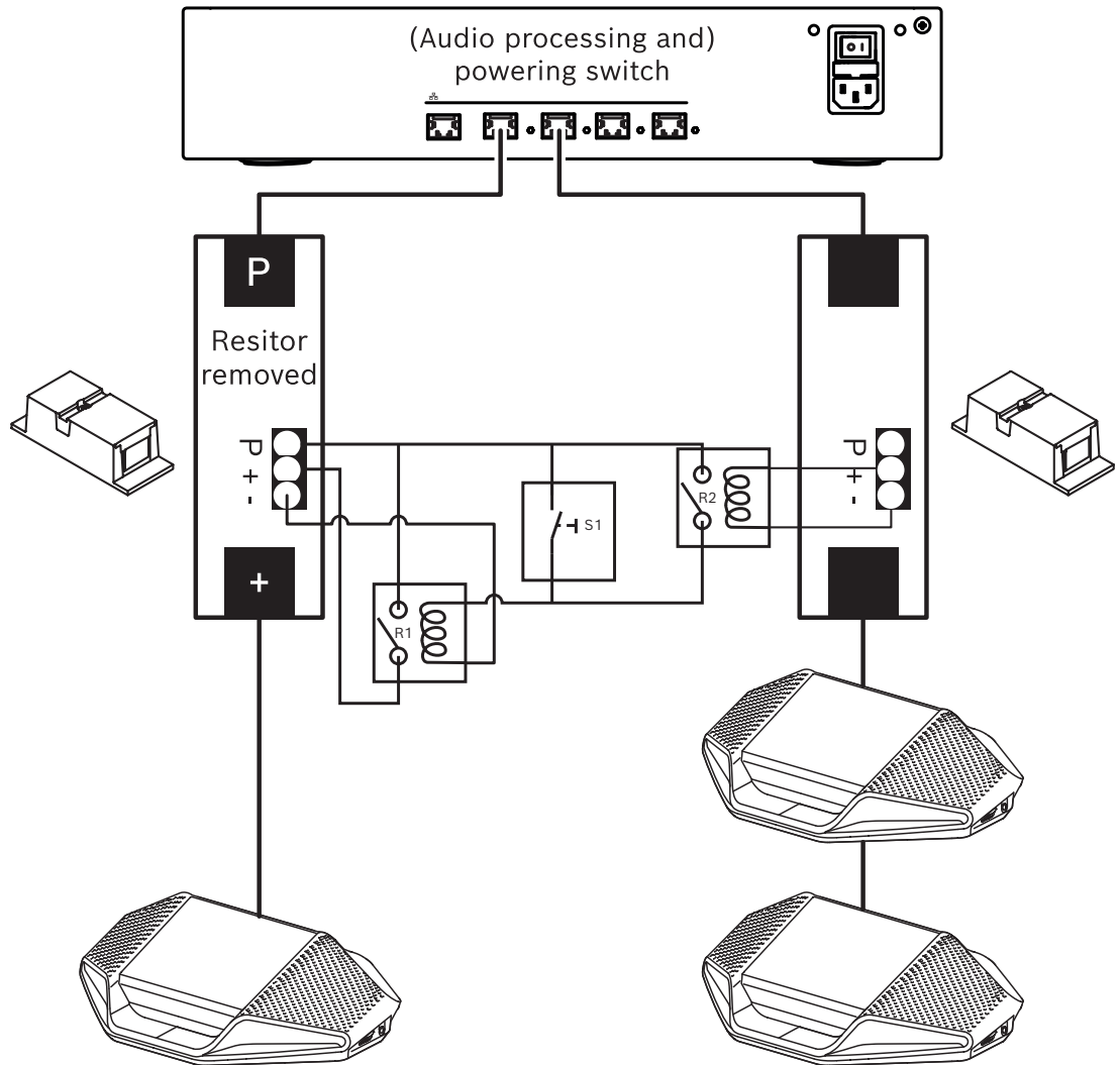
그림 5.8: 케이블 커플러와 사용자 제작 스위치를 사용하여 웨이크업 스위치 만들기 개략적인 작동 방식은 다음과 같습니다.
