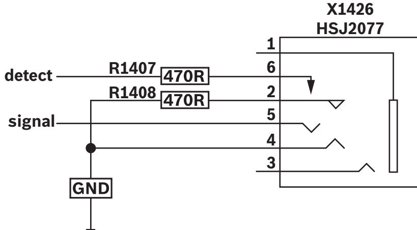
그림 7.13: 외부 헤드폰 커넥터 다이어그램
