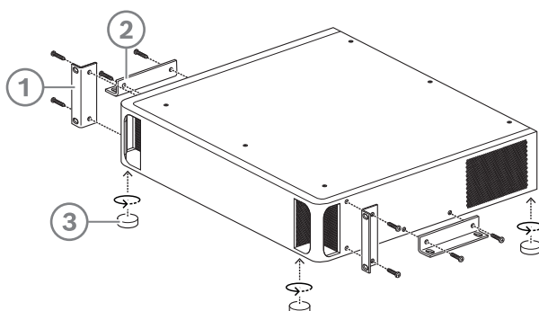
그림 6.4: 19인치 랙, 평평한 표면 및 피트 장착
