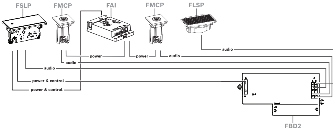
그림 7.21: 2개의 마이크가 있고 버튼이 없는 연단 좌석
