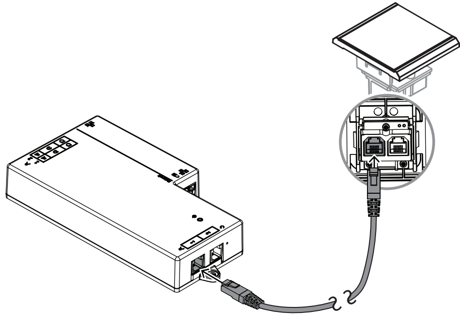
그림 7.19: DCNM-FIDP를 제어용 DCNM-FBD2에 연결
