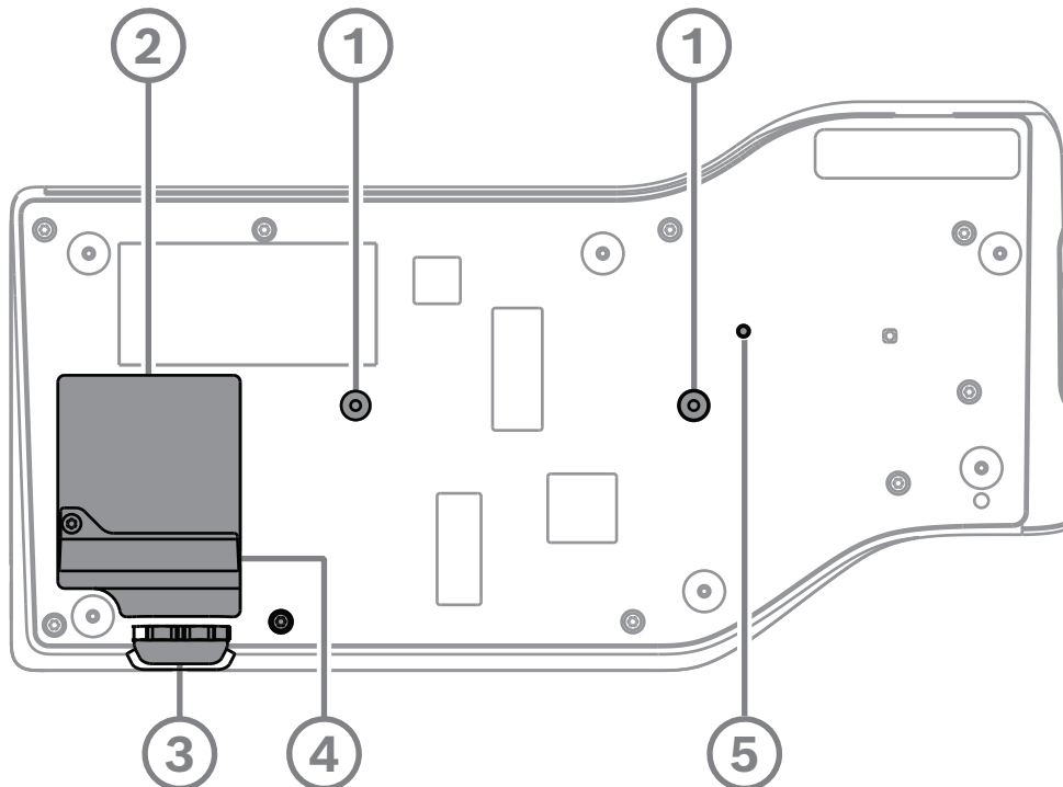
그림 7.3: DICIENTIS 회의 장치(DCNM-MMD / DCNM-MMD2) 하단면
