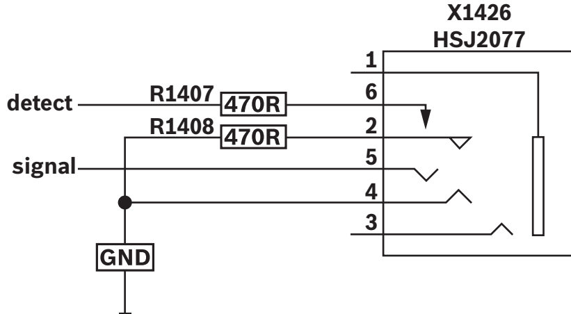
그림 7.23: 외부 헤드폰 커넥터 다이어그램
