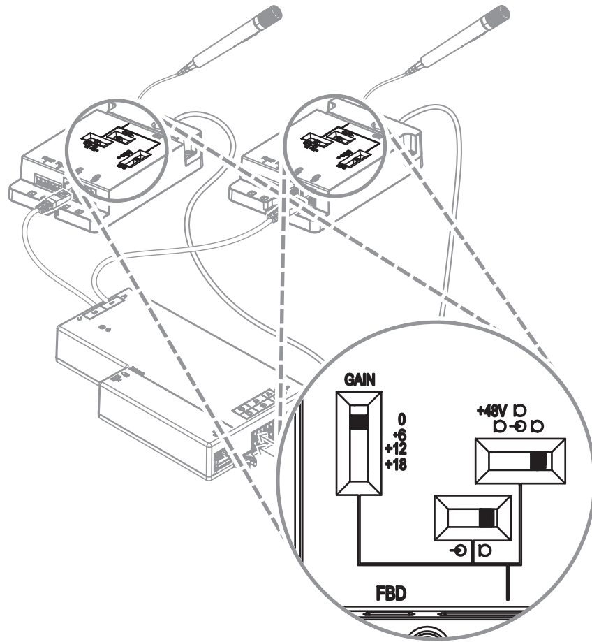
그림 7.18: DCNM-FHH/DCNM-FHHC 연결을 위한 DCNM-FAI 스위치 설정
