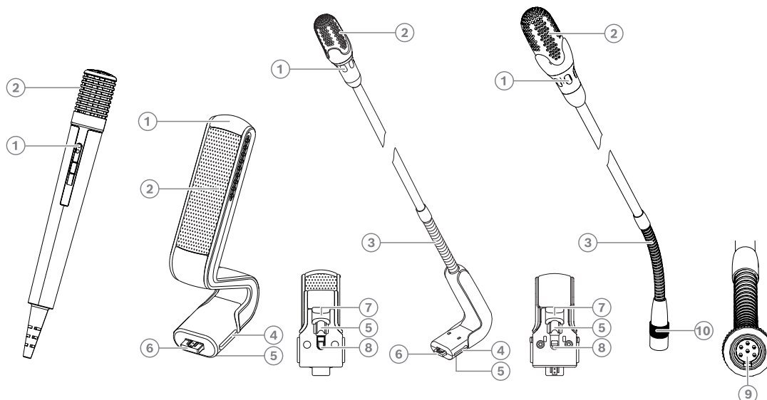
그림 7.26: DCNM-FHH/DCNM-FHHC, DCNM-HDMIC, DCNM-MICS/DCNM-MICL, DCNM-MICSLL/DCNM-MICSLs
