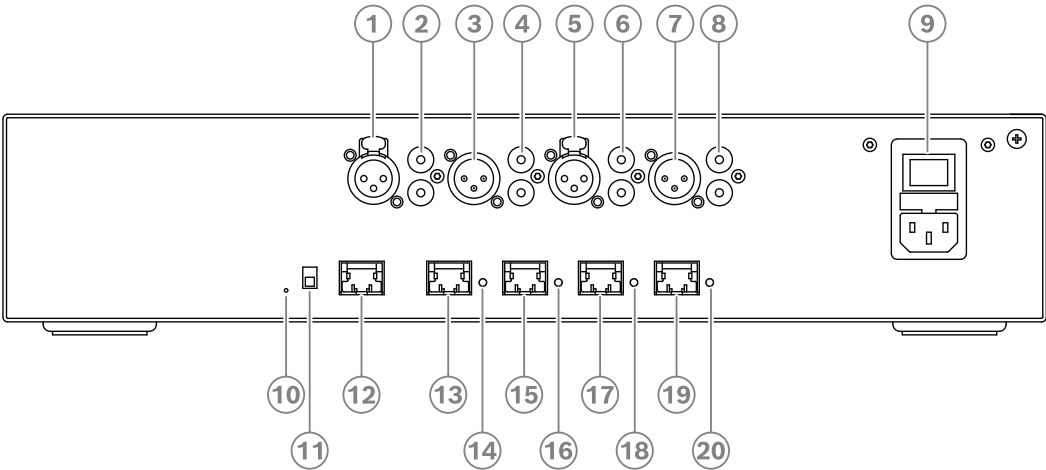
그림 6.2: 오디오 프로세서 및 파워링 스위치
