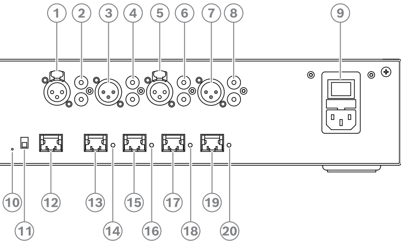
그림 4.2: 오디오 프로세서 및 파워링 스위치
