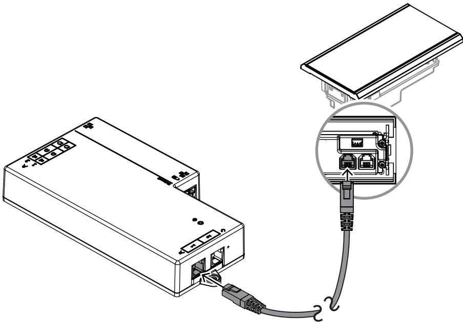
그림 7.7: DCNM-FVP를 제어용 DCNM-FBD2에 연결
