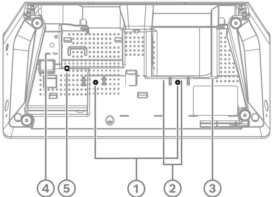
그림 7.25: DCNM-IDESK / DCNM-IDESKVID 하단면
