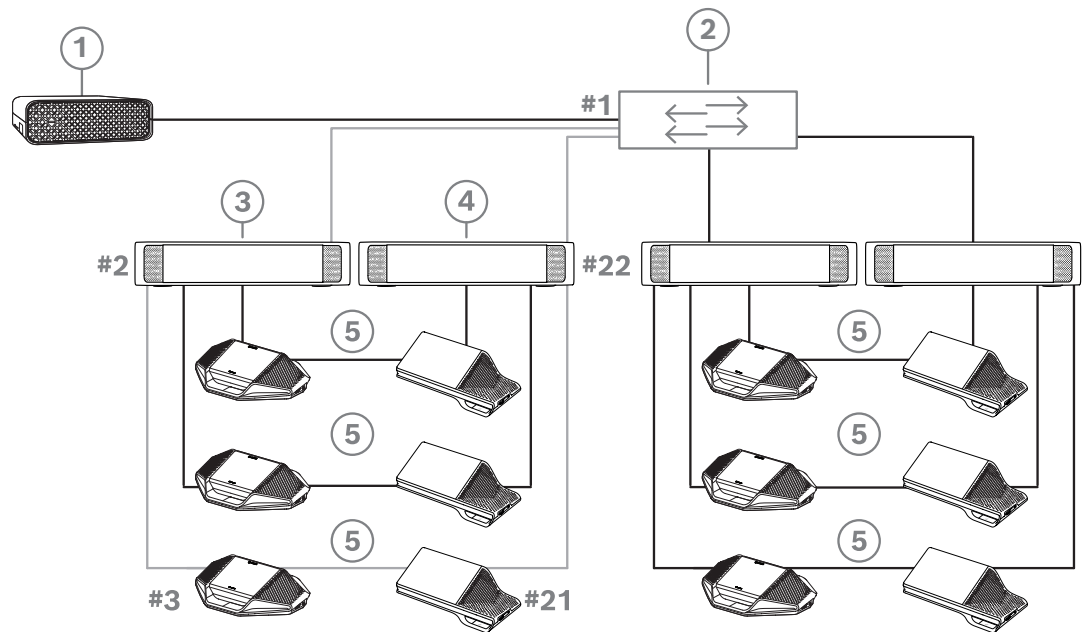
그림 4.9: DCNM-PS2 / DCNM-APS2 유형 장치 사이에서 리던던트 케이블로 연결된 DICENTIS 회의 장치
