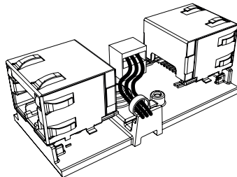
그림 5.6: 장력 해제 부위를 만들면 타이 랙이 전원 케이블이 뽑히는 것을 방지해줍니다.
