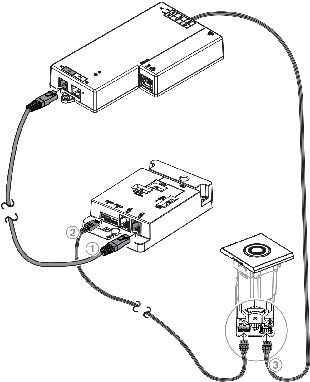
그림 7.15: DCNM-FAI를 통해 DCNM-FMCP를 DCNM-FBD2에 연결
