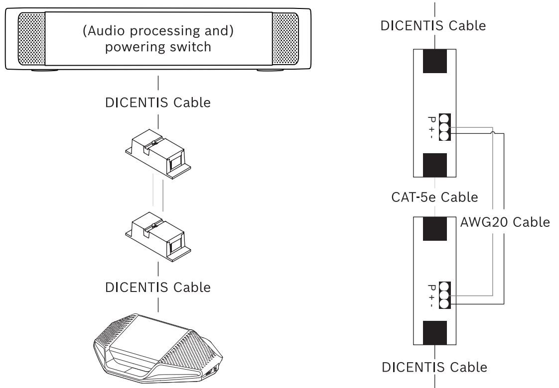
그림 5.3: 인터페이스로 사용된 케이블 커플러
