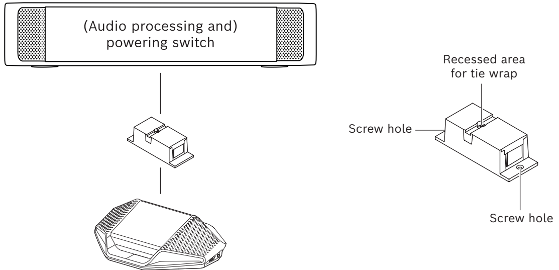
그림 5.2: 플로어 포드에 브레이크아웃 박스로 설치
