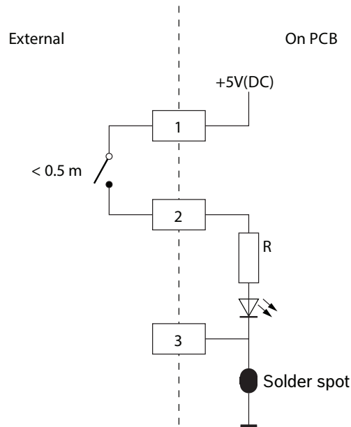
그림 7.11: 외부 접점, 연결 (2)
