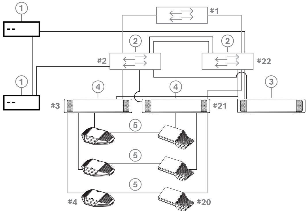
그림 4.10: 리던던트 구성요소 및 케이블이 있는 리던던트 DICENTIS 서버 PC
