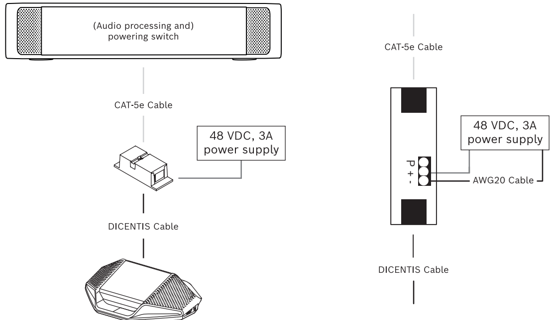
그림 5.5: 케이블을 통한 전력 공급
