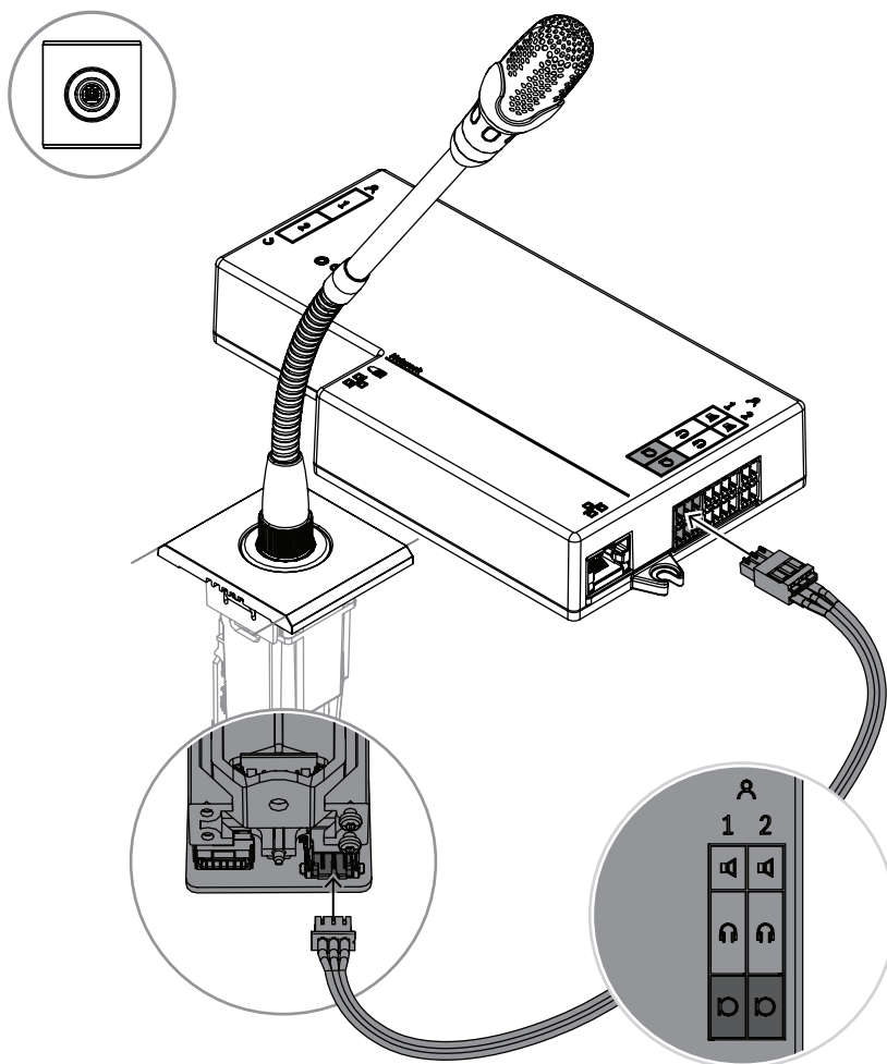
그림 7.5: DCNM-FBD2에 DCNM-FMCP 연결
