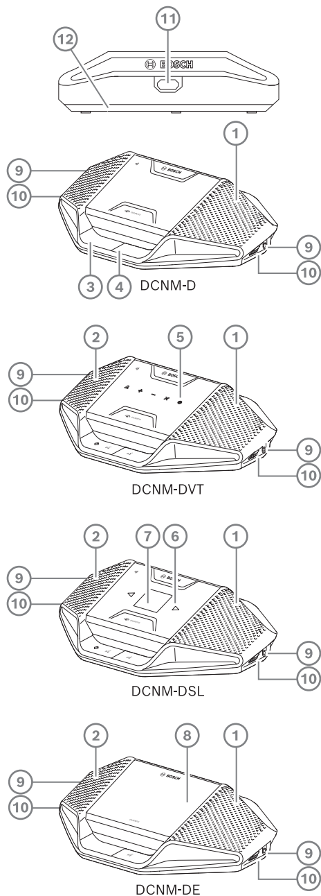
그림 7.2: 전면, 상단면, 후면, 측면
