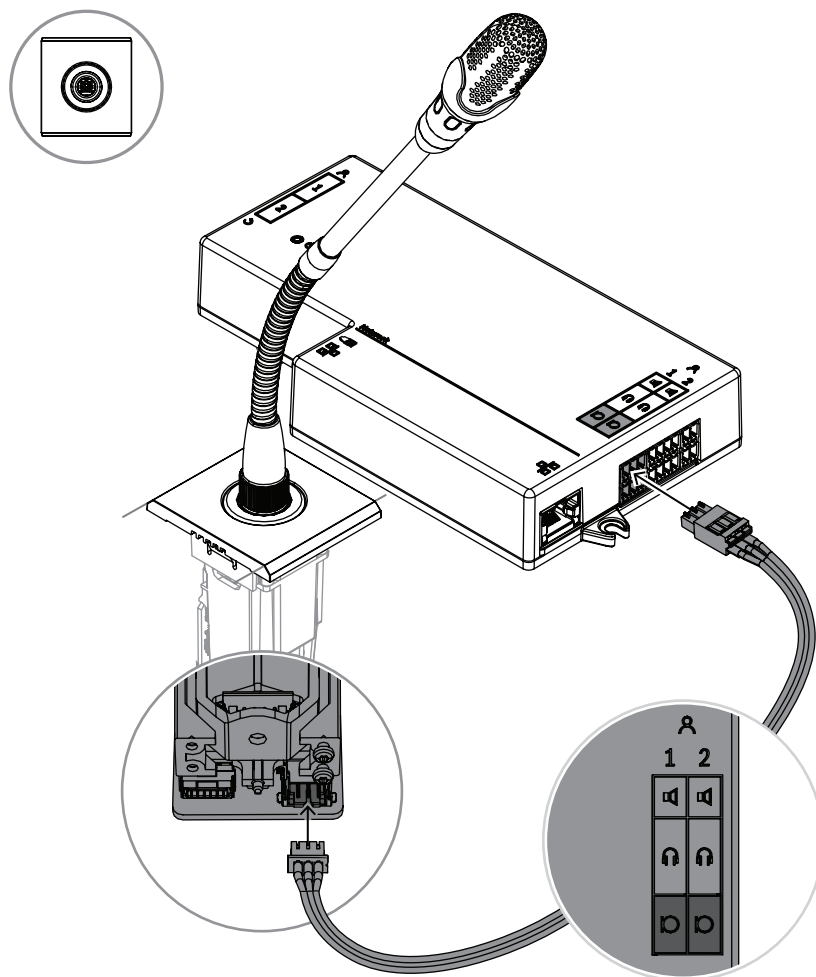
图片 7.5: 将DCNM-FMCP连接到DCNM-FBD2
