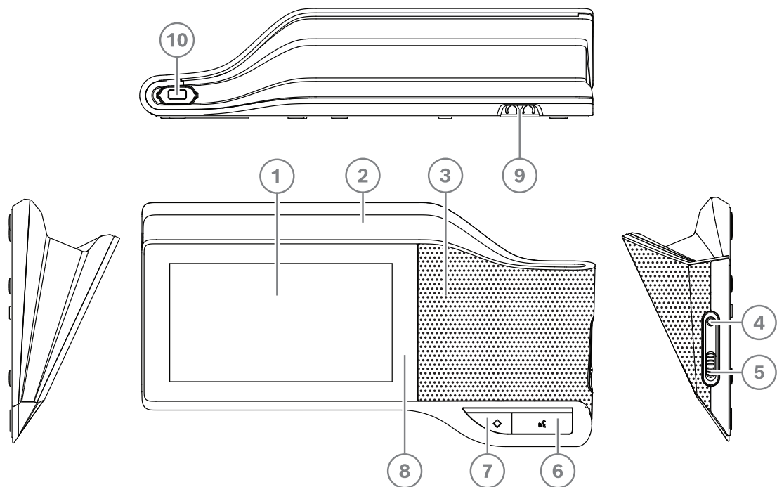
图片 7.1: 前视图、俯视图、后视图和侧视图
