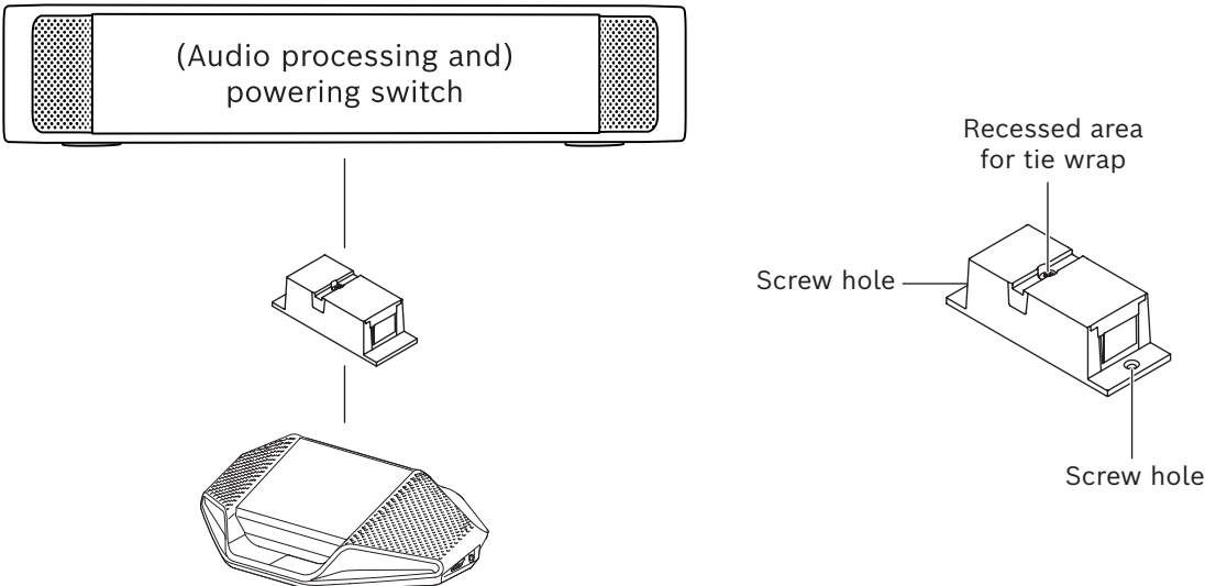
图片 5.2: 在地面箱中作为接线盒安装
