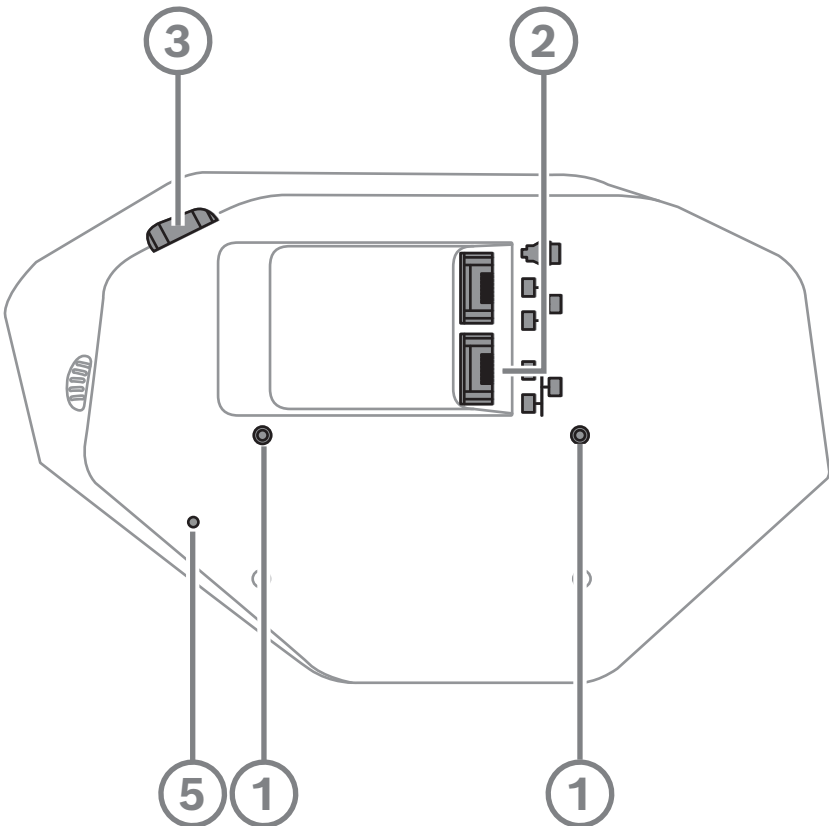
图片 7.4: 底视图DICENTIS设备(DCNM-D/DCNM-DVT/DCNM-DSL/DCNM-DE)
