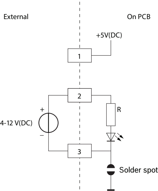
图片 7.10: 外部触点、连接 (1)
