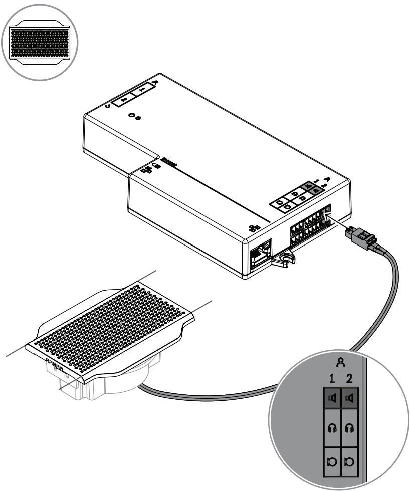
图片 7.6: 将一个DCNM-FLSP连接到DCNM-FBD2
