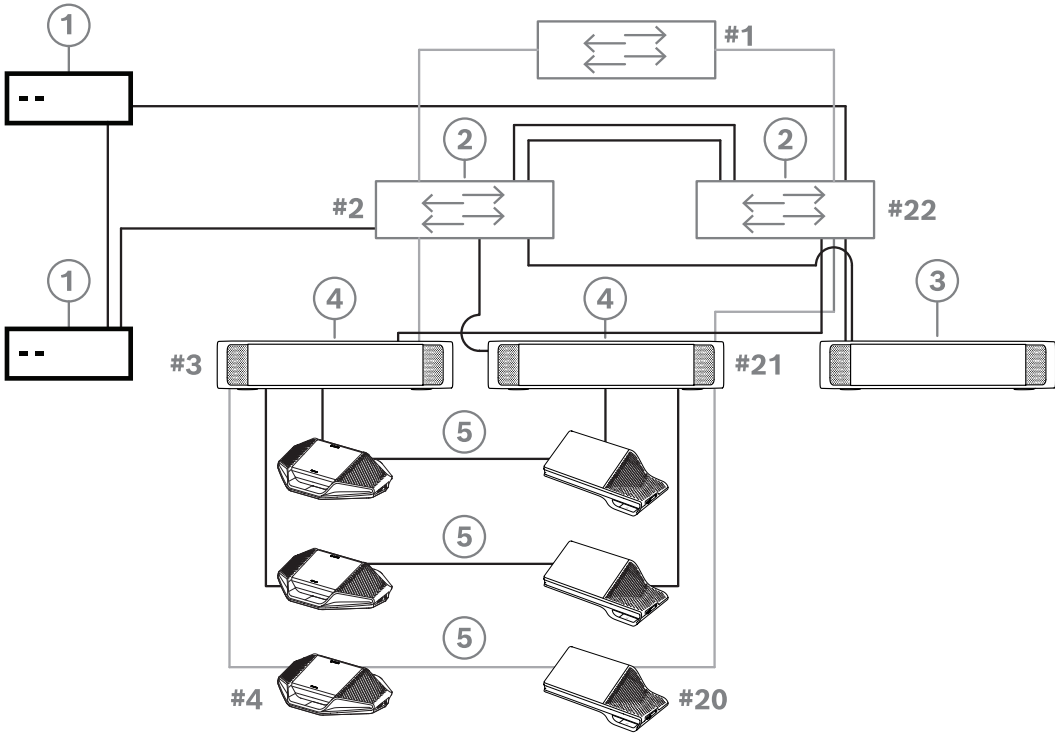
图片 4.10: 具有冗余组件和电缆的冗余DICENTIS服务器PC
