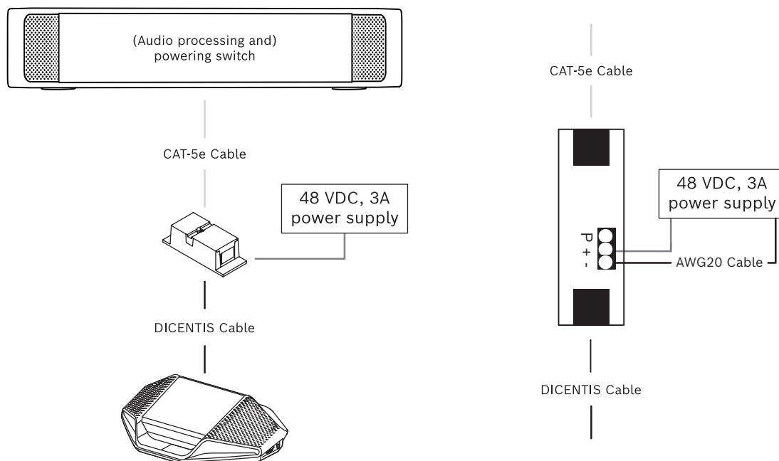
图片 5.5: 通过电缆供电
