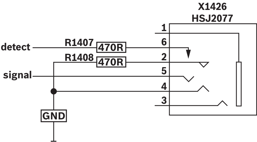
图片 7.13: 外部耳机连接器图
