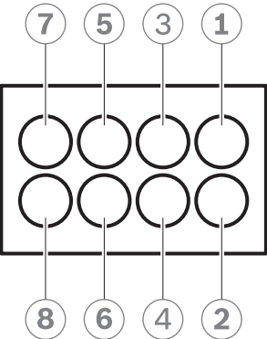
图片 5.14: 8针Phoenix连接器
