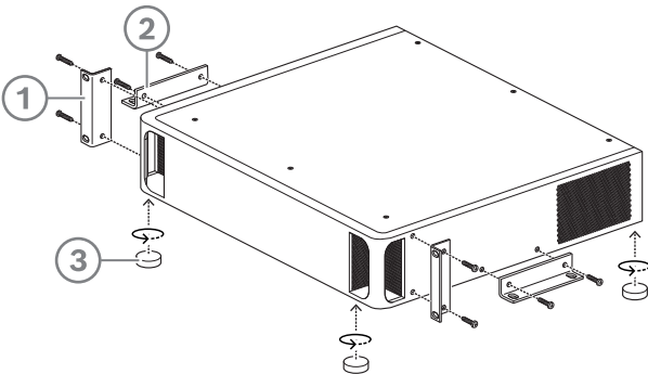
图片 6.4: 19英寸机柜、平坦的表面和支脚安装
