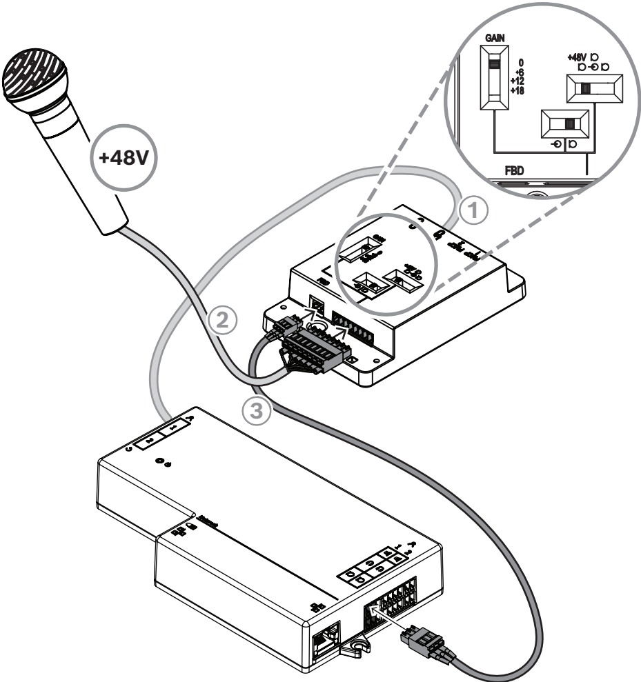
图片 7.16: 通过DCNM-FAI将幻象电源话筒连接到DCNM-FBD2
