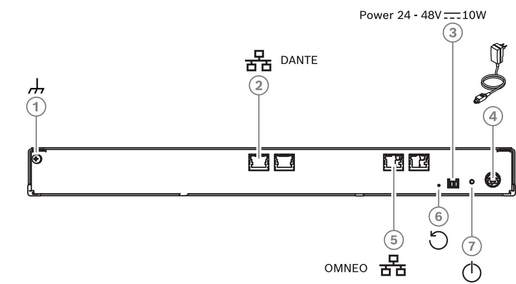
图片 6.5: OMN-DANTEGTW后面板说明
