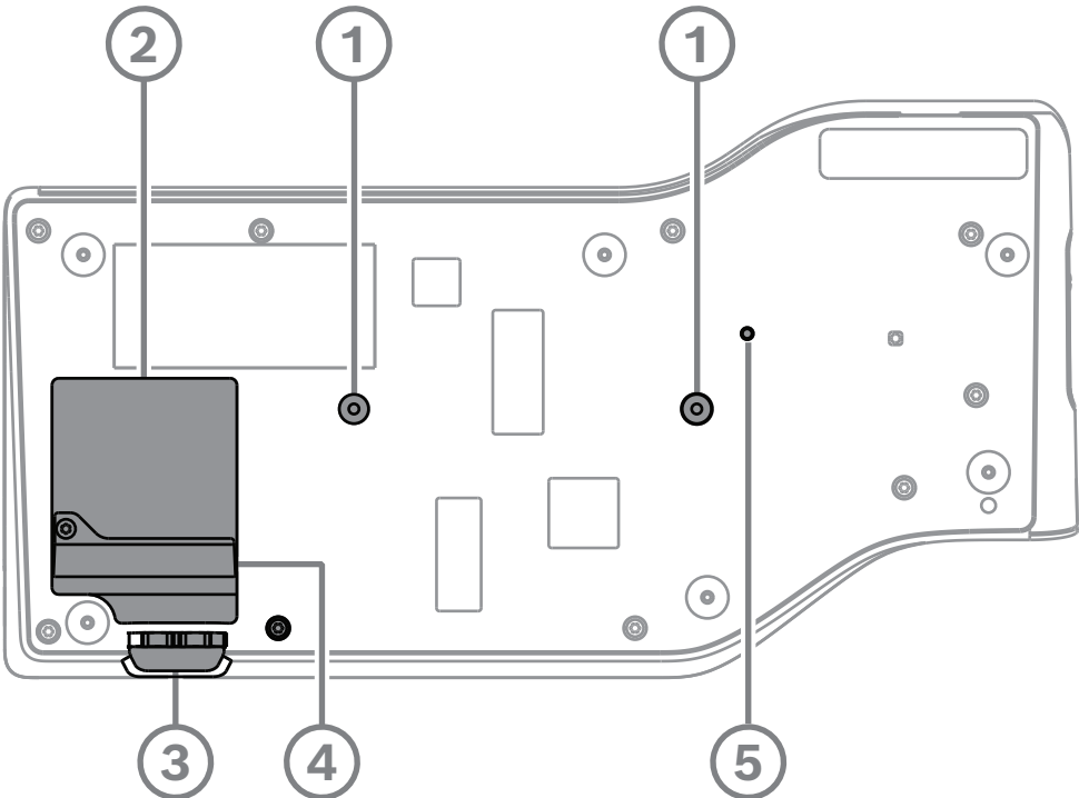
图片 7.3: 底视图讨论DICENTIS设备(DCNM-MMD/DCNM-MMD2)
