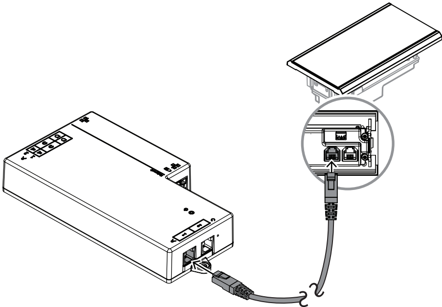
图片 7.7: 将DCNM-FVP连接到DCNM-FBD2以进行控制
