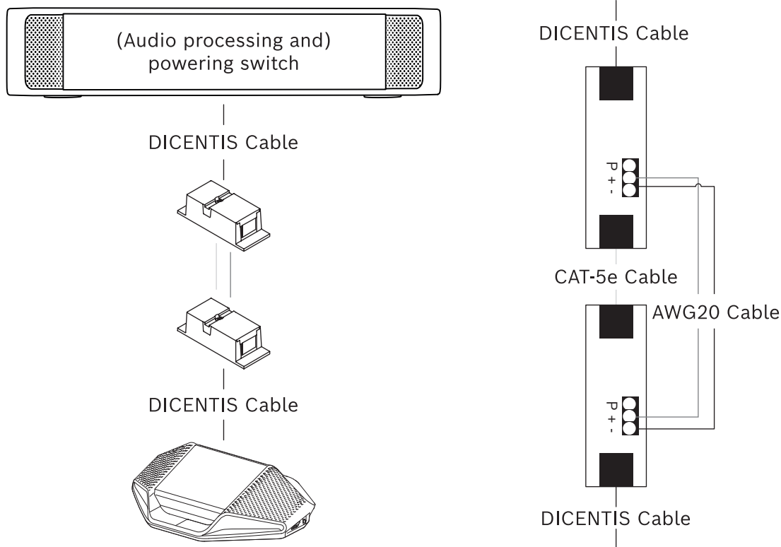
图片 5.3: 用作接口的电缆耦合器
