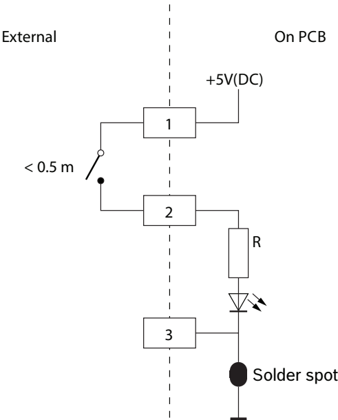
图片 7.11: 外部触点，连接 (2)
