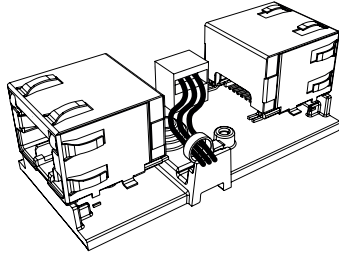
图片 5.7: 释放一下张力，绑带可防止电源线被意外拔出。
