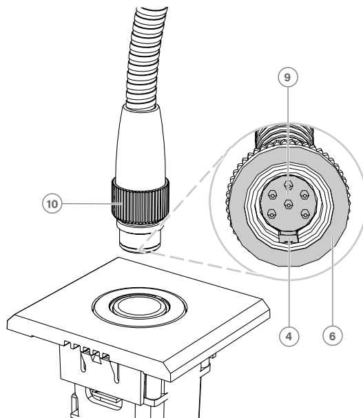
图片 7.28: DCNM-MICSL/DCNM-MICSL连接
