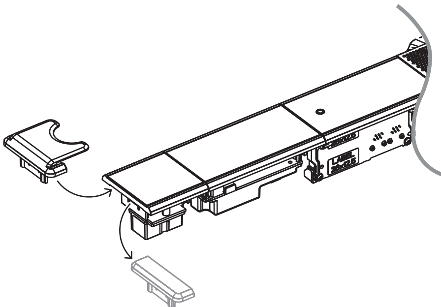
图片 7.20: 用DCNM-FICH替换DCNM-FEC
