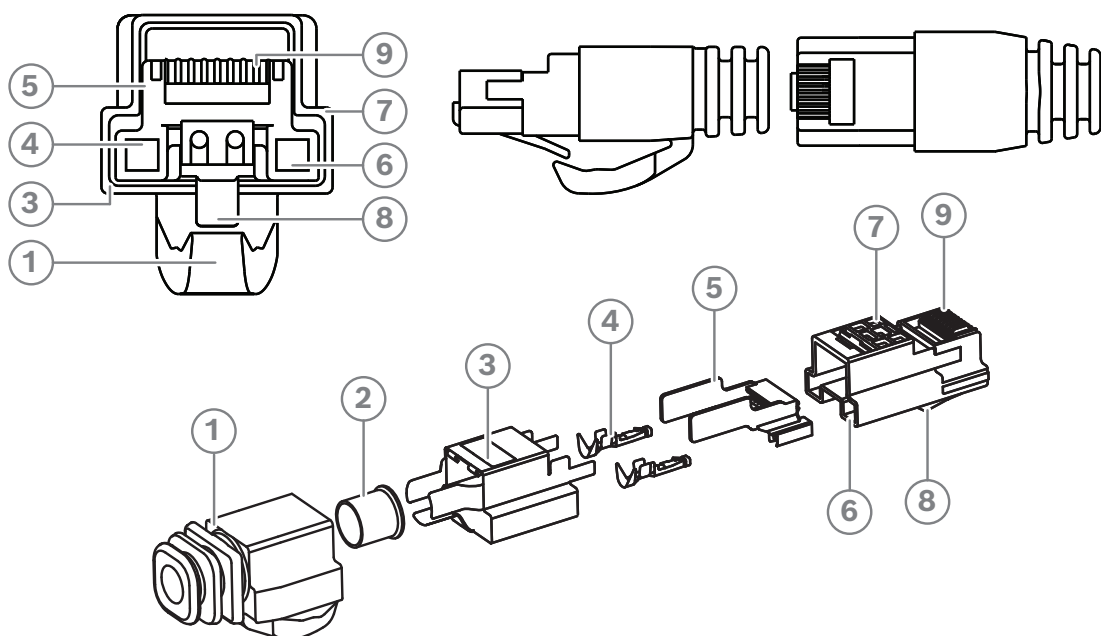
图片 5.10: DCNM-CBCON前视图和分解视图
