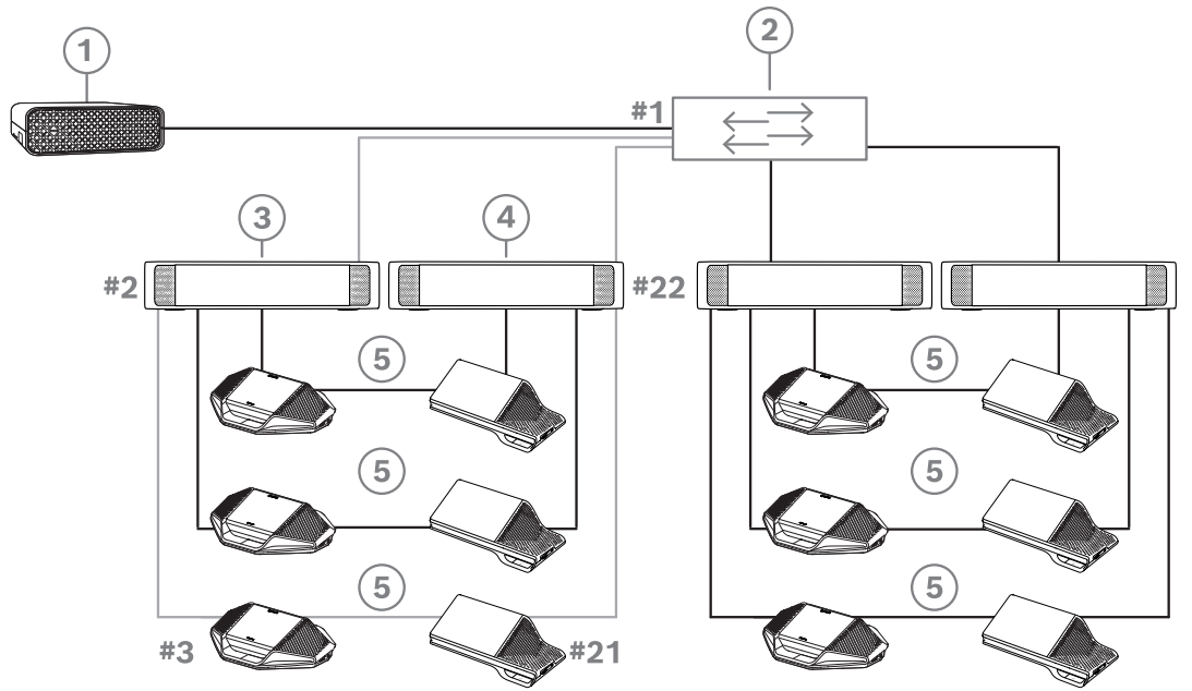
图片 4.9: 与DCNM-PS2和DCNM-APS2型装置之间的冗余布线连接的DICENTIS讨论设备
