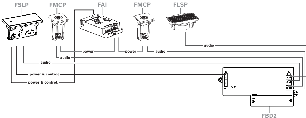
图片 7.21: 配两个话筒且无按钮的讲台席位
