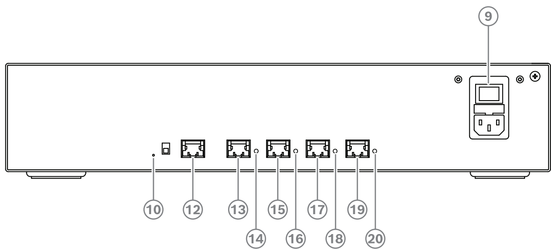
图片 4.3: 供电交换机
