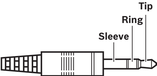
图片 7.14: 耳机插孔连接
