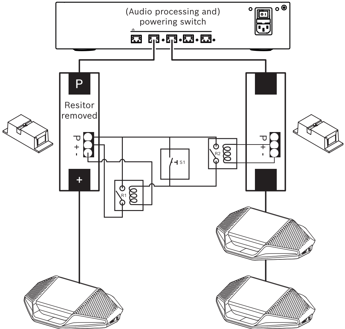
图片 5.8: 使用电缆耦合器和定制开关制作唤醒开关
