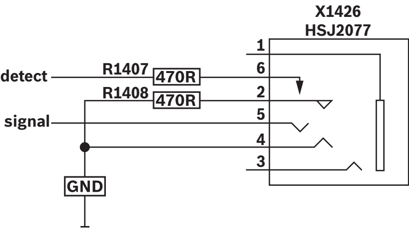
图片 7.23: 外部耳机连接器图
