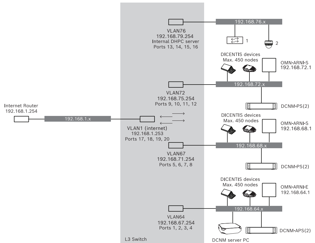
图片 3.3: 典型的多子网DICENTIS会议系统
