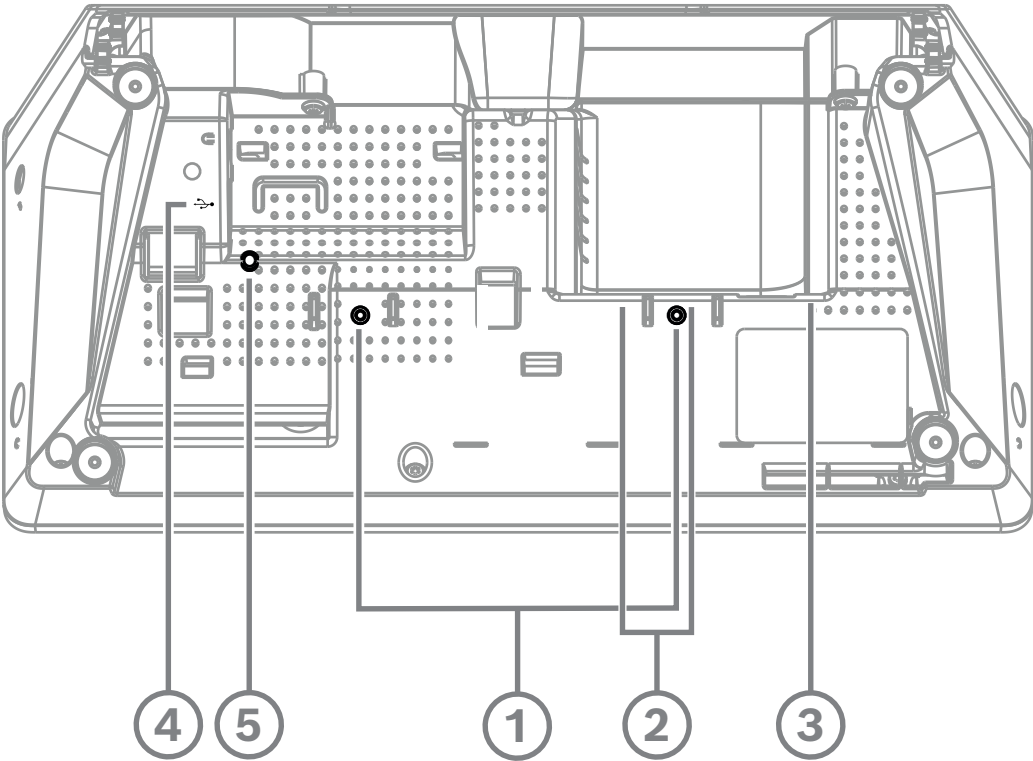
图片 7.25: DCNM-IDESK/DCNM-IDESKVID底视图
