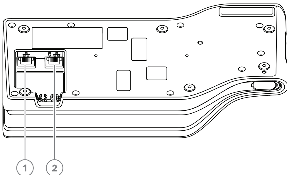
图片 4.6: 底视图DICENTIS设备(DCNM-MMD/DCNM-MMD2)
