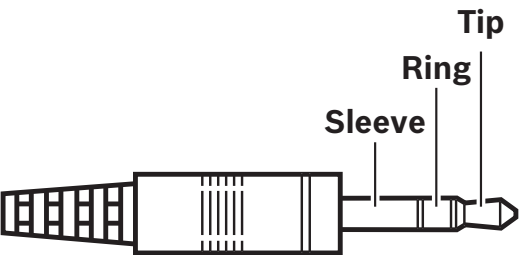
图片 7.24: 耳机插孔连接
