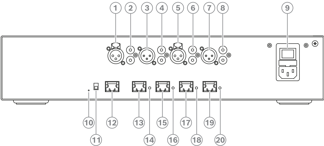
图片 4.2: 音频处理器兼供电交换机
