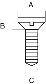
图片 5.13: 螺丝最大直径
