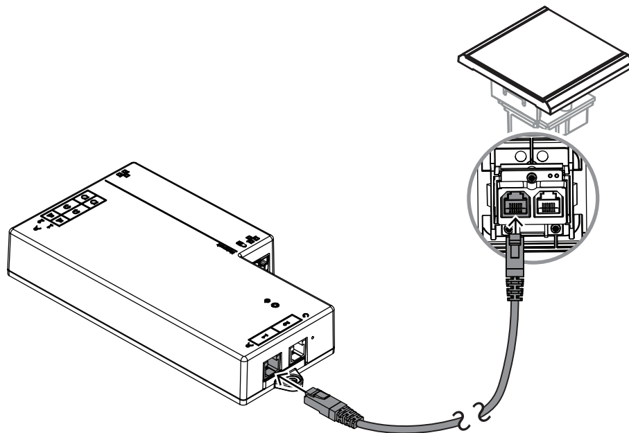
图片 7.19: 将DCNM-FIDP连接到DCNM-FBD2以进行控制
