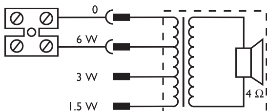
Abb. 3: Schaltbild
