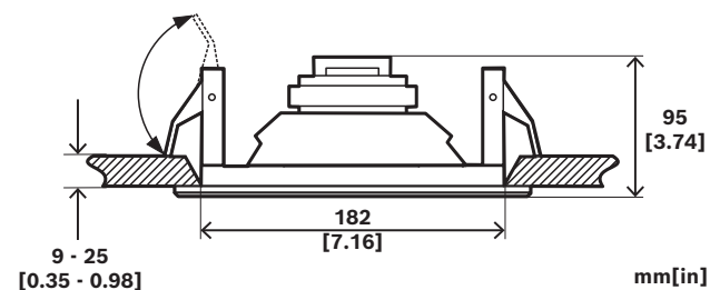
Abb. 2: Abmessungen (in mm)
