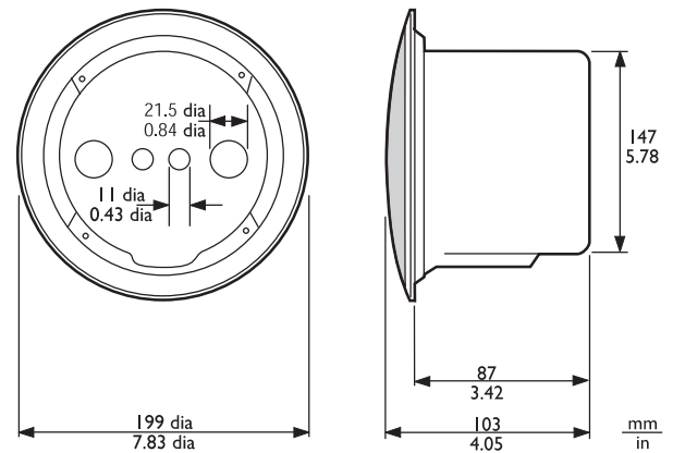
Abb. 8: LBC3090/01 + LBC3080/01 Feuerschutzhaube, Abmessungen in mm
