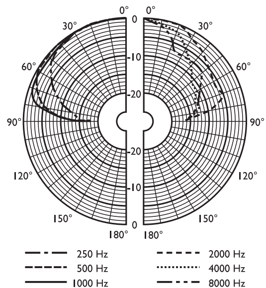
Abb. 5: Polardiagramm (gemessen mit rosa Rauschen)
