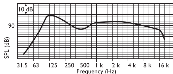
Rys. 4: Charakterystyka przenoszenia
