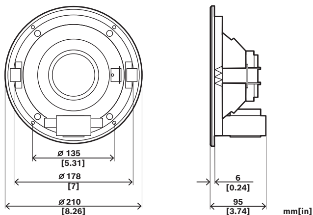
Rys. 1: Wymiary w mm
