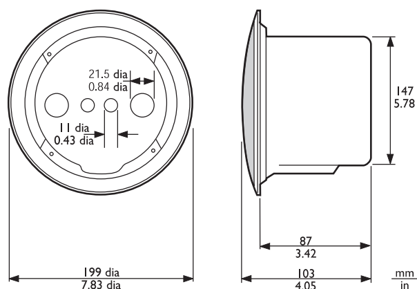
Rys. 8: Głośnik LBC3090/01 z osłoną przeciwpożarową LBC3080/01 – wymiary w mm
