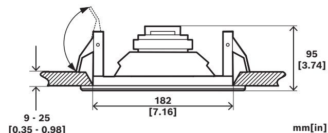
Rys. 2: Wymiary w mm
