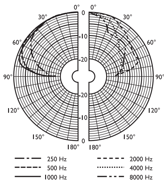
Rys. 5: Charakterystyka kierunkowości (pomiar z użyciem szumu różowego)
