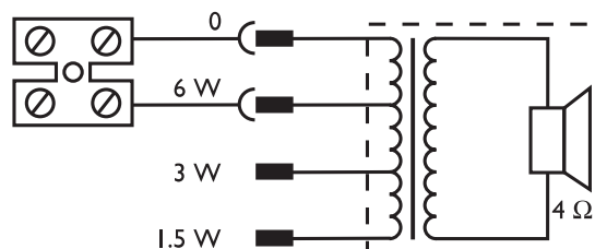
Rys. 3: Schemat elektryczny
