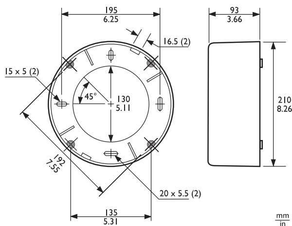
Rys. 7: Wymiary w mm
