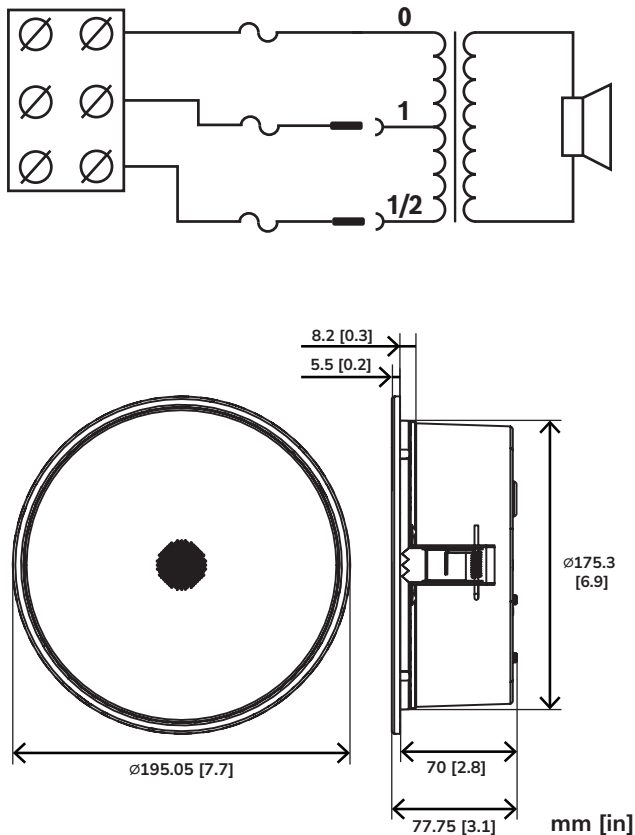
Fig. 1: Dimensions
