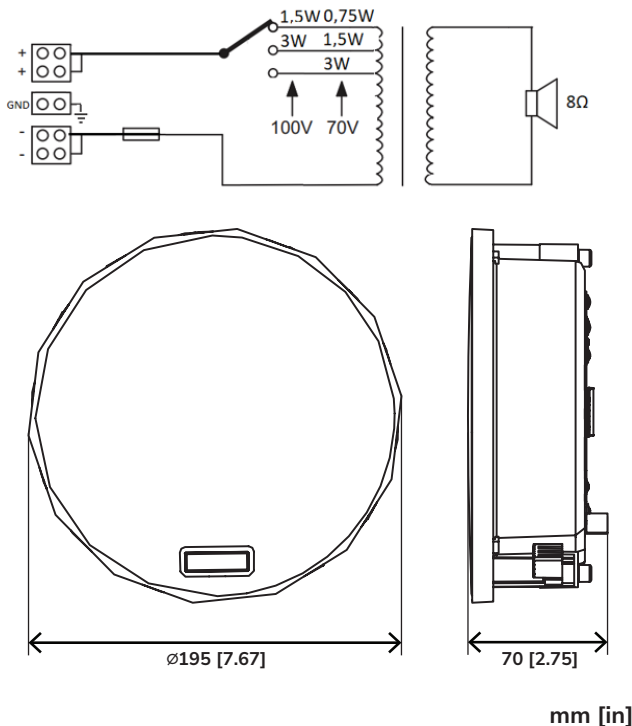
Fig. 1: Dimensions
