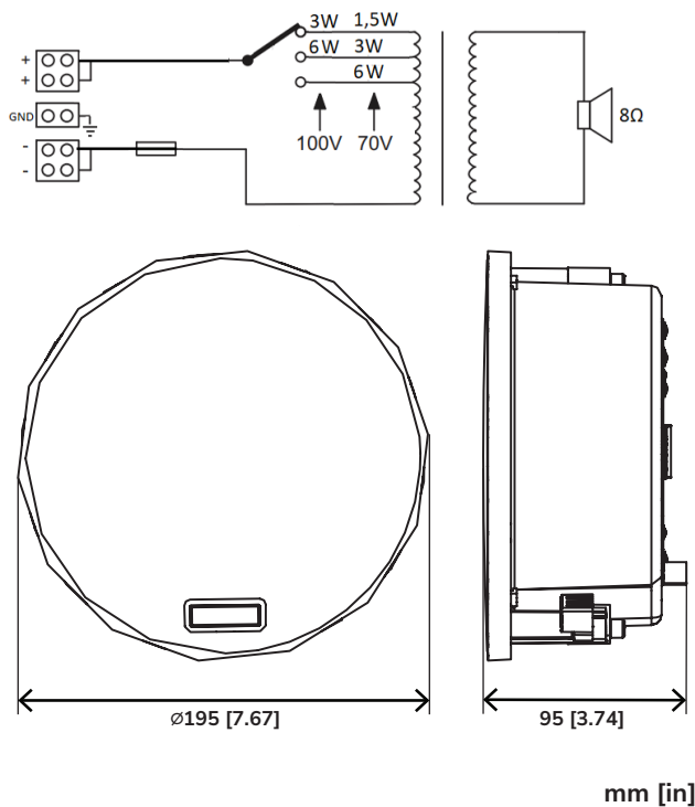
Fig. 1: Dimensions
