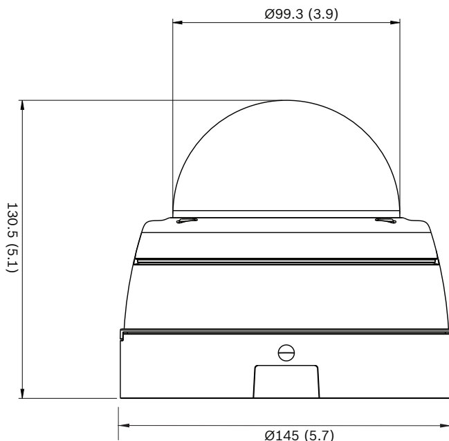
Рис. 1: Размеры (мм/дюймы)
