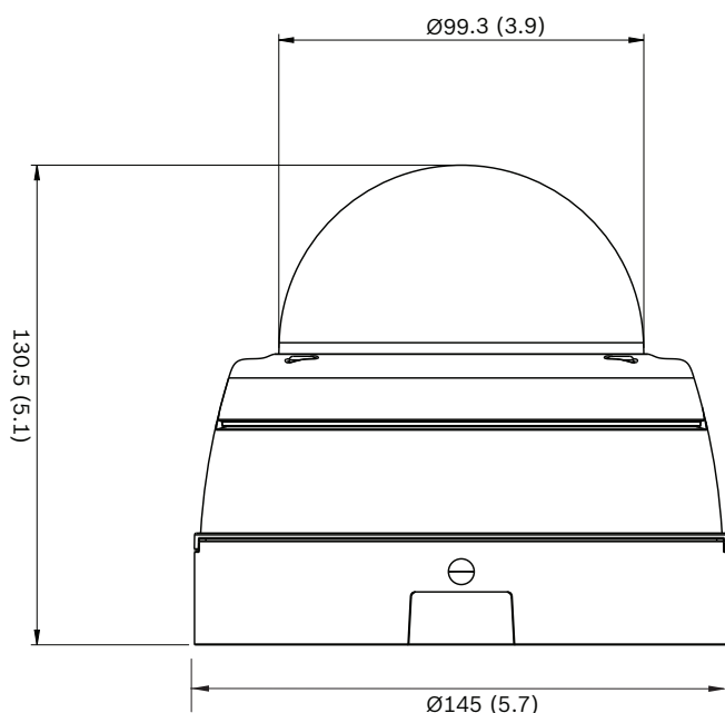
图片 1: 尺寸, 单位为毫米 (英寸)
