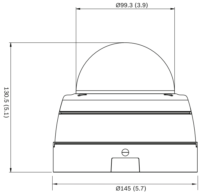
그림 1: 크기 (mm(인치))
