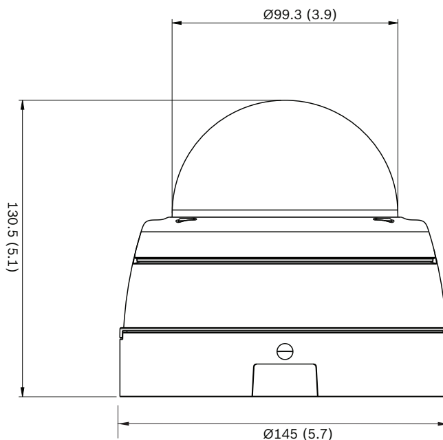
Fig. 1: Mått mm (tum)
