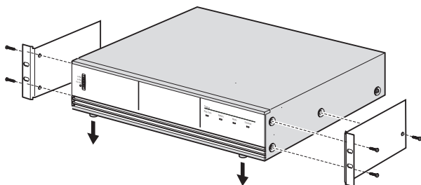
Figura 4.1: Staffe per montaggio in rack da 19"
