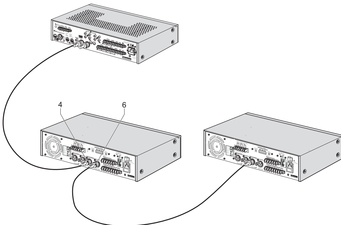
Figura 6.2: Ingresso di linea e collegamento Loop-Through
