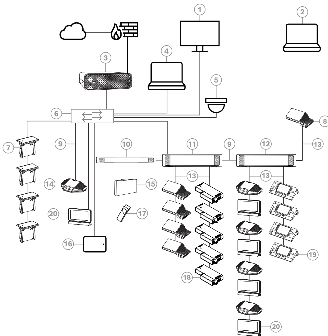
Figura 3.1: Configuración típica del sistema de conferencias DICENTIS
