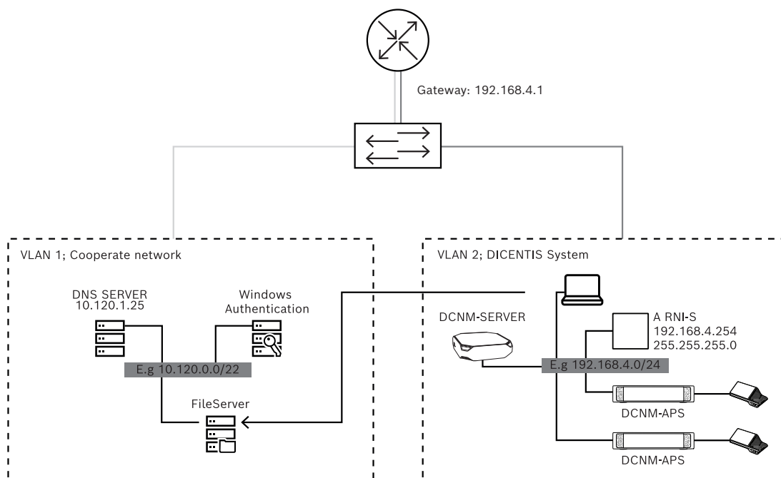
Figura 5.2: Diagrama del sistema
