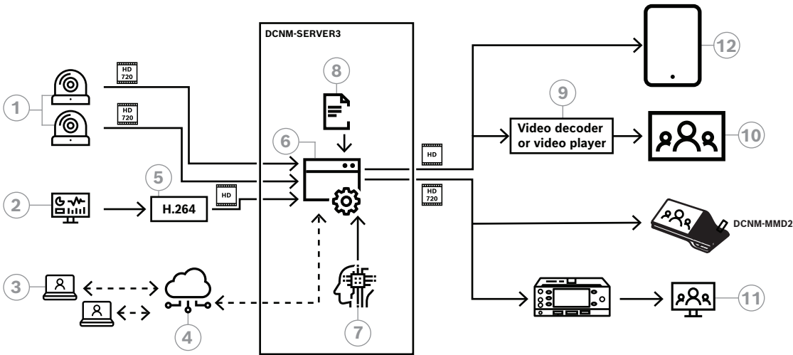
Figura 8.2: Gateway de mídia – diagrama conceitual
