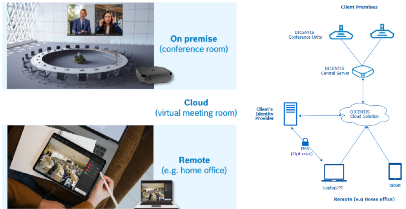
Figura 7.1: Integração do SSO com a solução Reuniões Híbridas DICENTIS
