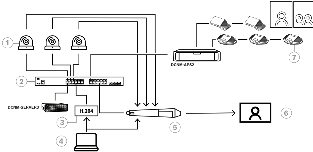
Şekil 8.4: SDI donanım değiştirme kullanan bağımsız DICIENTIS sistemi
