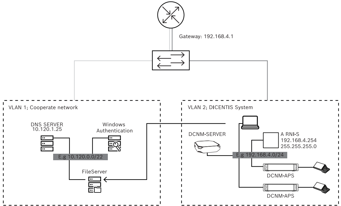
Şekil 5.2: Sistem şeması
