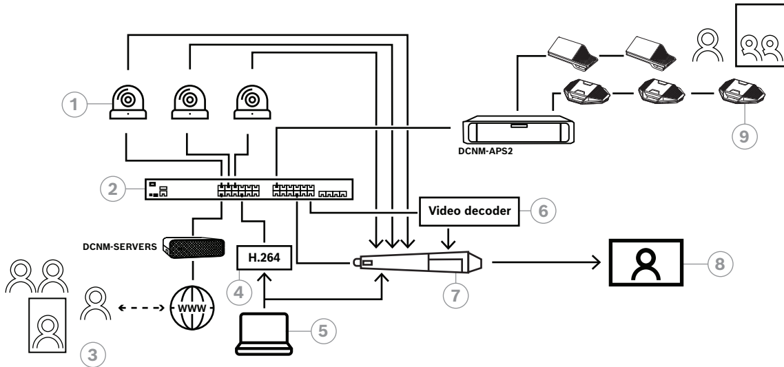
Şekil 8.6: SDI donanım değişirme kullanan DICENTIS hibrit toplantılar
