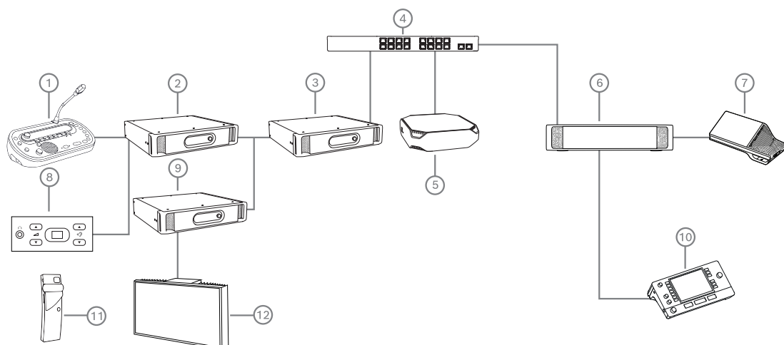
圖片 5.8: 連接 DICENTIS 與 DCN NG
