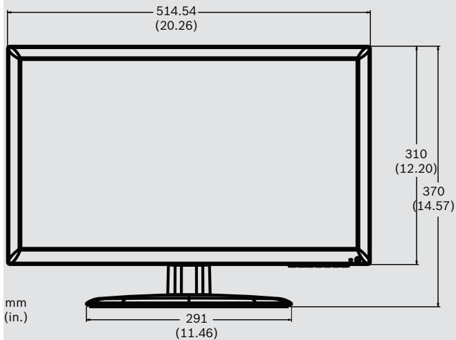
UML-223-90: Vooraanzicht
