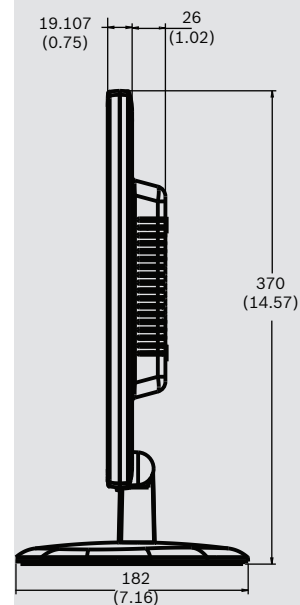
UML-223-90: Zijaanzicht
