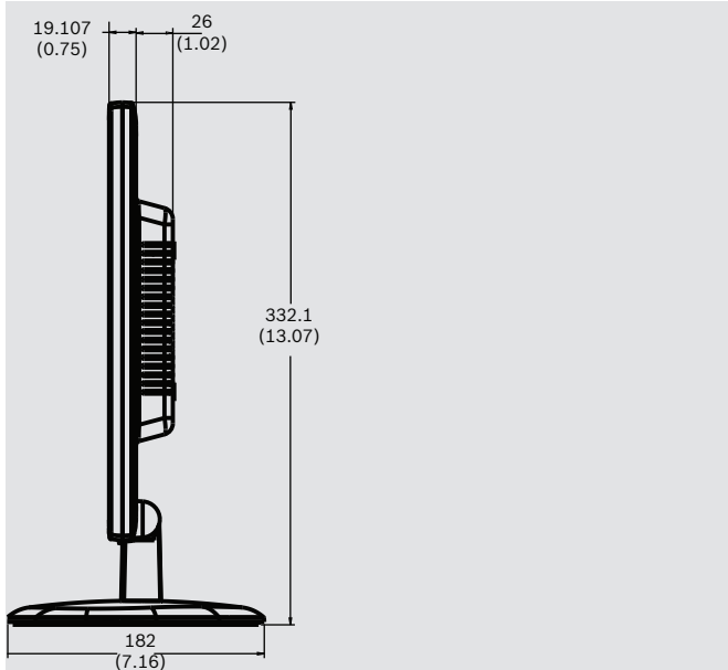
UML-193-90: Zijaanzicht
